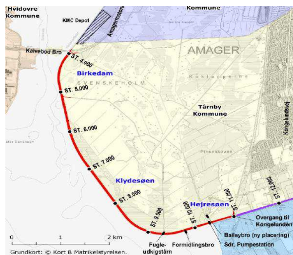
Figur 21: Plantegning af hævnig af Vestamager Kystdige, 2012.
