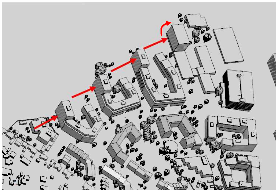
Figur 9-8 Illustration af vind fra vest, der møder de høje bygninger mod nord. Hjørnehvirvel antydnet for den nordligste bygning, men kan opstå ved alle fire høje bygninger. (Bilag 6 – vindvurdering)
