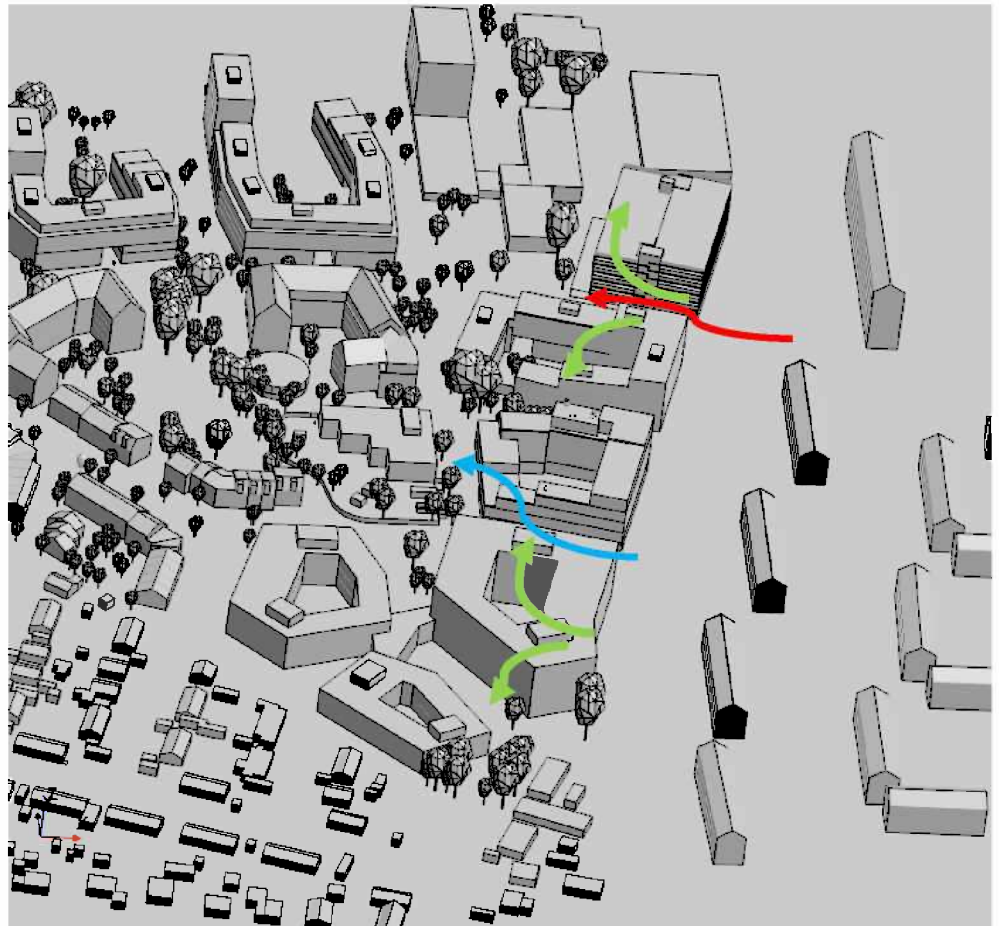
Figur 9-6 Område med potentiel vindforstærkning, illustration af vind over en bygning (blå pil), vind rundt om hjørnerne i gadeplan (rød pil) og vind langs facaderne (grøn pil). (Bilag 6 vindvurdering)
