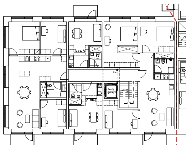
Boligplaner 1-3 sal
