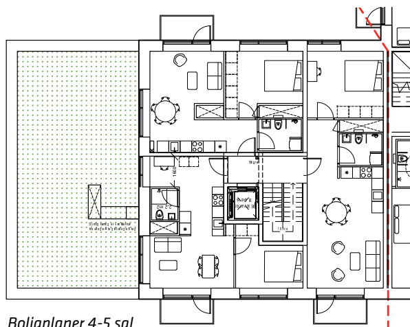
Boligplaner 4-5 sal
