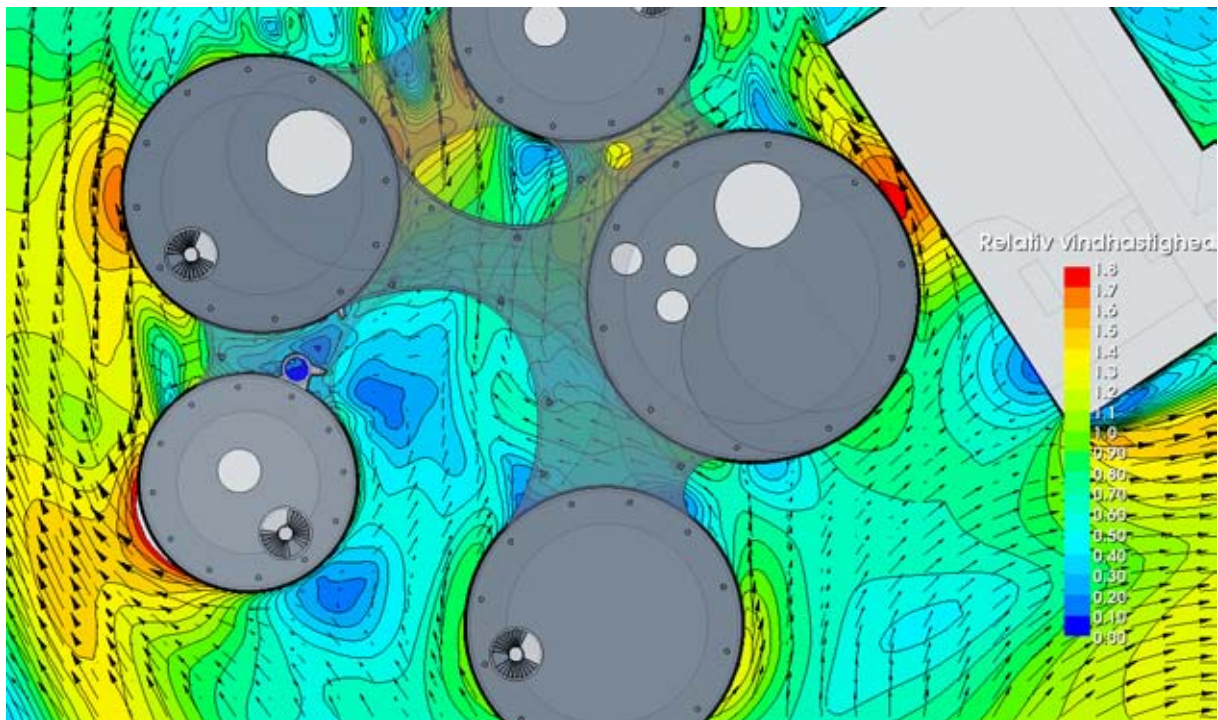
Figur 6.16 Konturer for relativ gust equivalent mean wind speed. Søndenvind. 1,5 m over det centrale terrasseområde mellem bygningerne. Nord opad.
