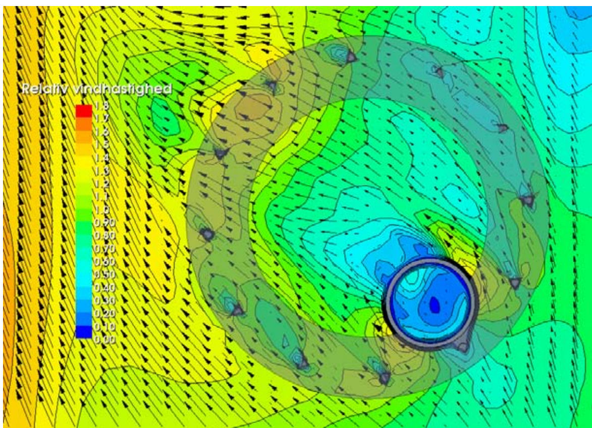
Figur 6.19 Konturer for relativ gust equivalent mean wind speed. Terrasse A. Sydvesten-vind. Nord opad.
