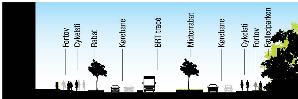
Figur 2. Principtværsnit af det midtlagte bustracé.
