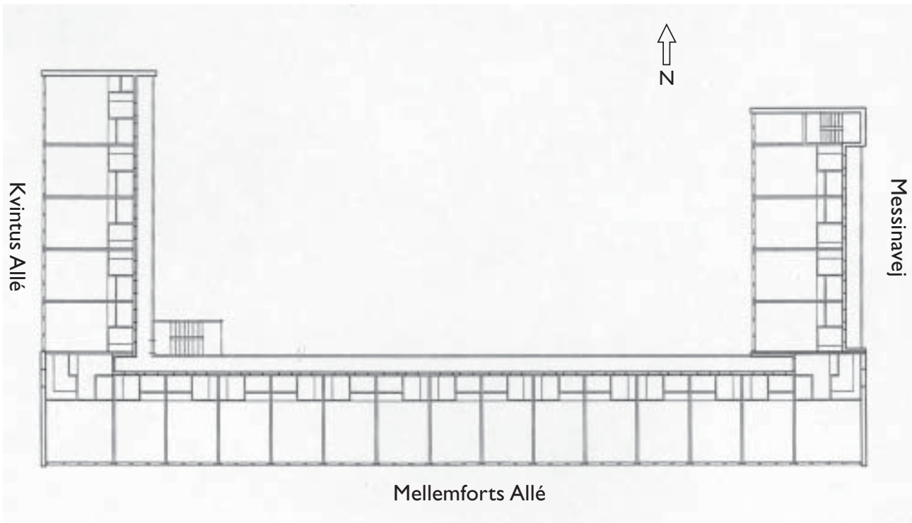
Plan af normaletage før og efter ombygning.
