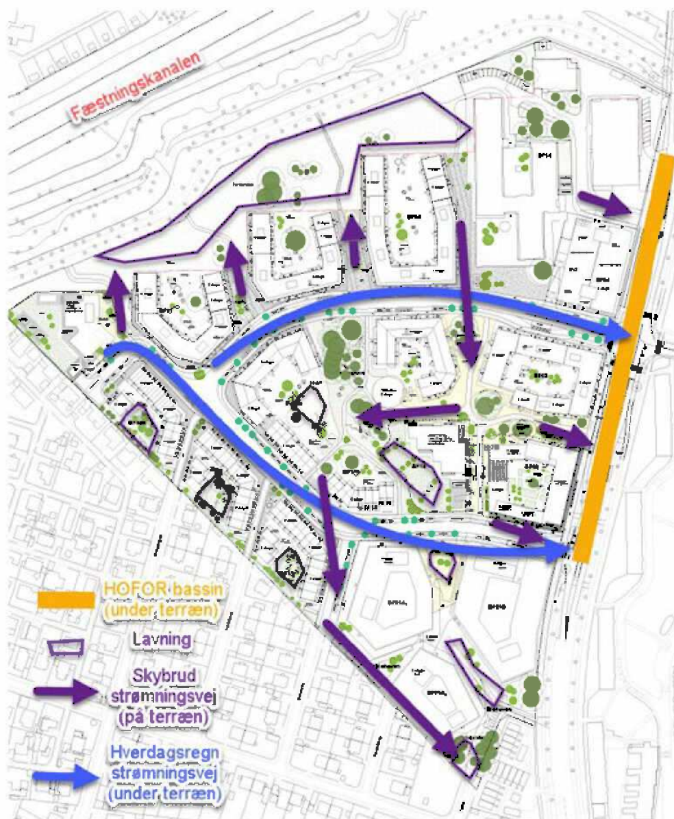
Figur 12-7 Principskitse med samlet løsningsforslag
