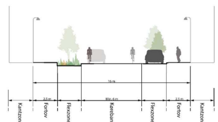
Figur 3: Tværrprofil for Bøjlevej
