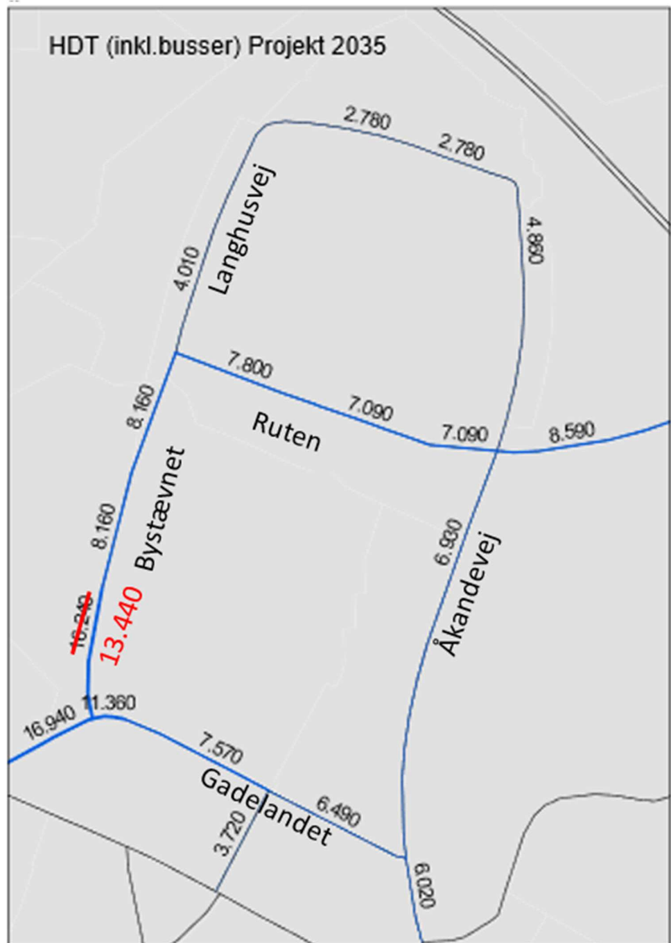
Figur 6: Beregnet hverdagsdøgntrafik, HDT, efter åbning mellem Tingbjerg og Husum 2035. "Kilde VVM-undersøgelsen" og Vejdirektoratets efterfølgende kommentering i mail af 6. april 2022
