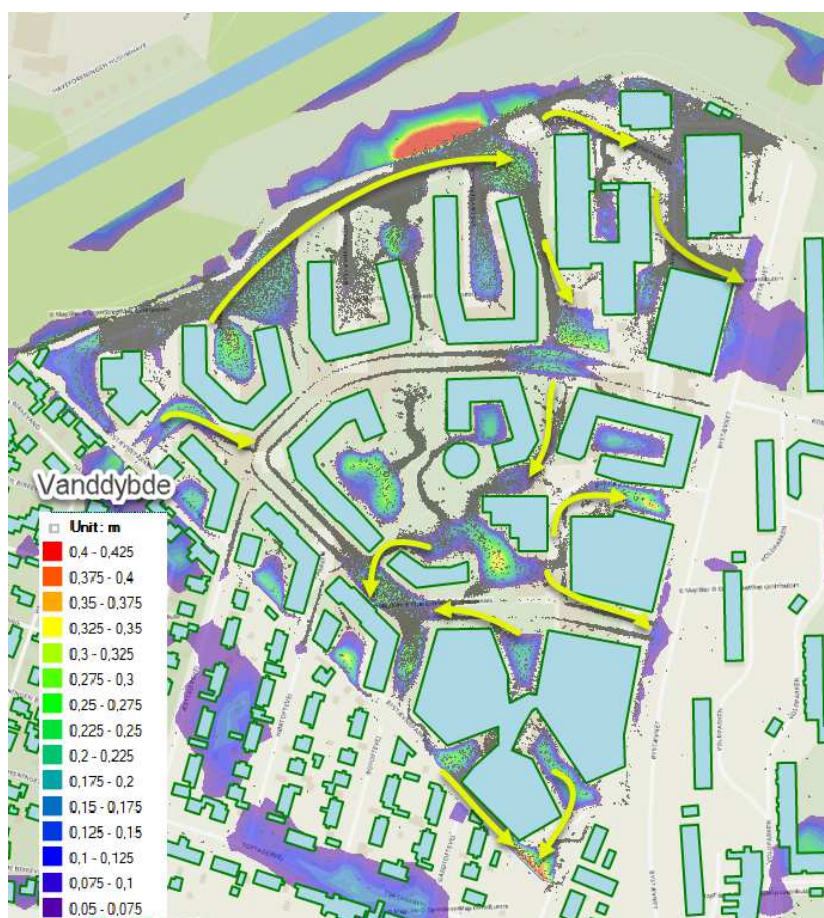
Figur 11 Vandets vej inden for Bystævneparken
