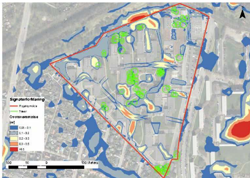
Figur 12-6 Overblik over træer og lavninger på Bystævneparken.
