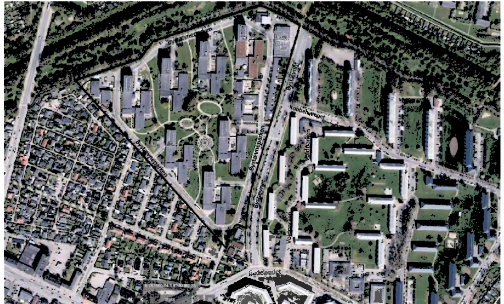
Figur 11-1 Bystævneparken oversigtskort
