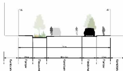
Figur 11-6 Tværprofil for Bøjlevej
