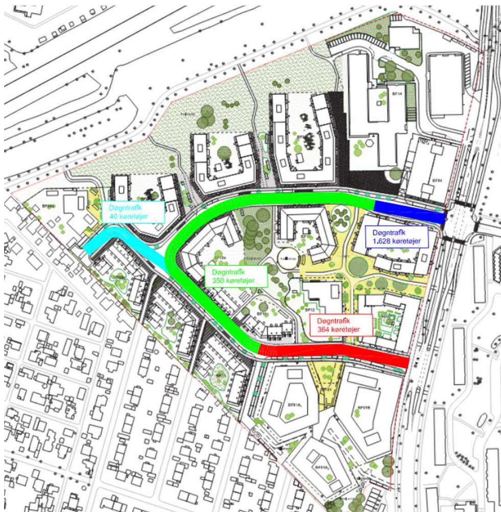
Figur 2: Den skønnede interne fordeling af trafikken, foretaget af COWI på baggrund af turrater fra Københavns Kommune. Trafiktallene er angivet som HDT i farvede sektioner; blå = 1628, grøn = 350, rød = 364, turkis = 40.
