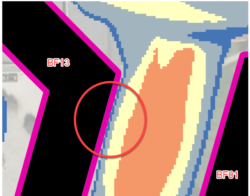
Figur 18: Detalje af oversvømmelse mellem BF13 og BF01, hvor der er lille overlap mellem 1-meter bufferzone og vanddybde på 5 cm ved BF13.
