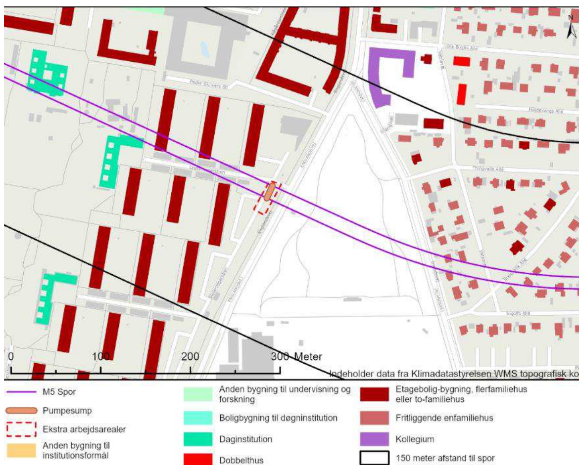
Figur 9-5 Omfanget af boliger og andre bebyggelser inden for 150 meter omkring sporerne ved det midlertidige arbejdsareal ved Lygtemagerstien.
