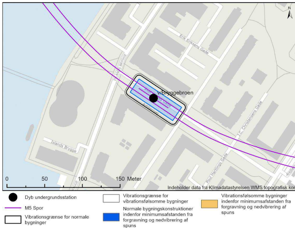
Figur 17-6 Vibrationskort for bygningsskadelige vibrationer ved etablering af byggegrubeindfatning ved forgravning og nedvibrering af spuns ved Bryggebroen (Bgb).
