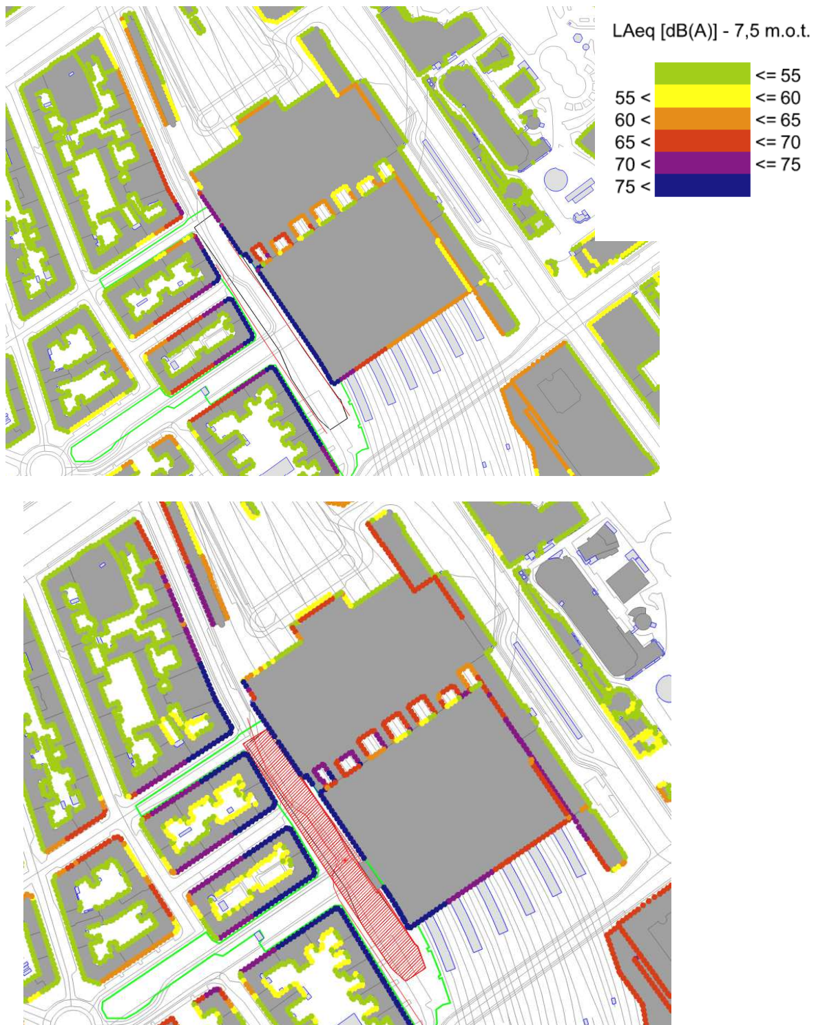
Figur 7-6 Øverst ses den beregnede støjdbredelse ved etablering af spurs, ved København H, som vil medføre en støjpåvirkning på 84 dB(A) på den nærmeste facade. Nederst er vist den beregnede støjdbredelse ved etablering af sekantpæle, som vil medføre en støjpåvirkning på 91 dB(A) på den nærmeste facade.
