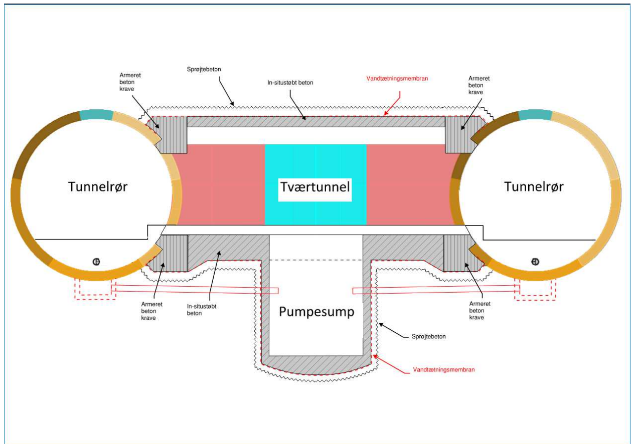
Figur 4-6 Tværsnit af en mulig udformning af en tværtunnel med pumpesump, der viser tværtunnelen mellem de to borede tunnelrør og selve pumpesumpen, der vil befinde sig under tunnelrørenes niveau.
