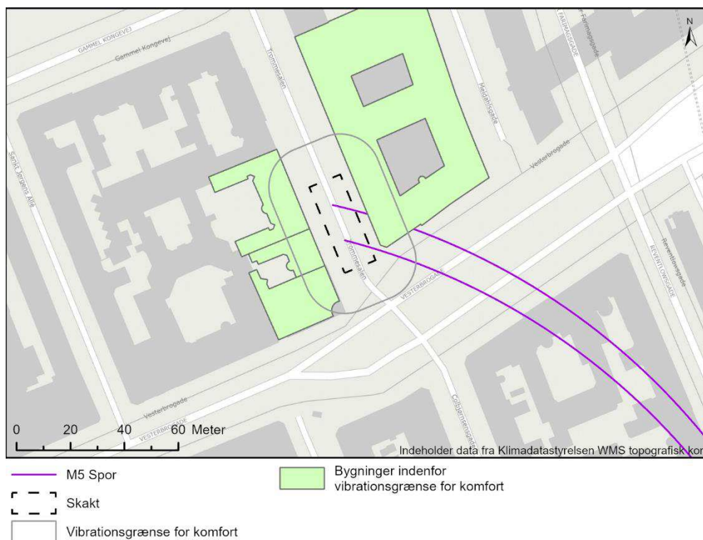
Figur 17-14 Vibrationskort for vibrationskomfort ved etablering af byggegrubeindfatning ved boring af sekantpæle ved Vesterbrogade (Vbg).
