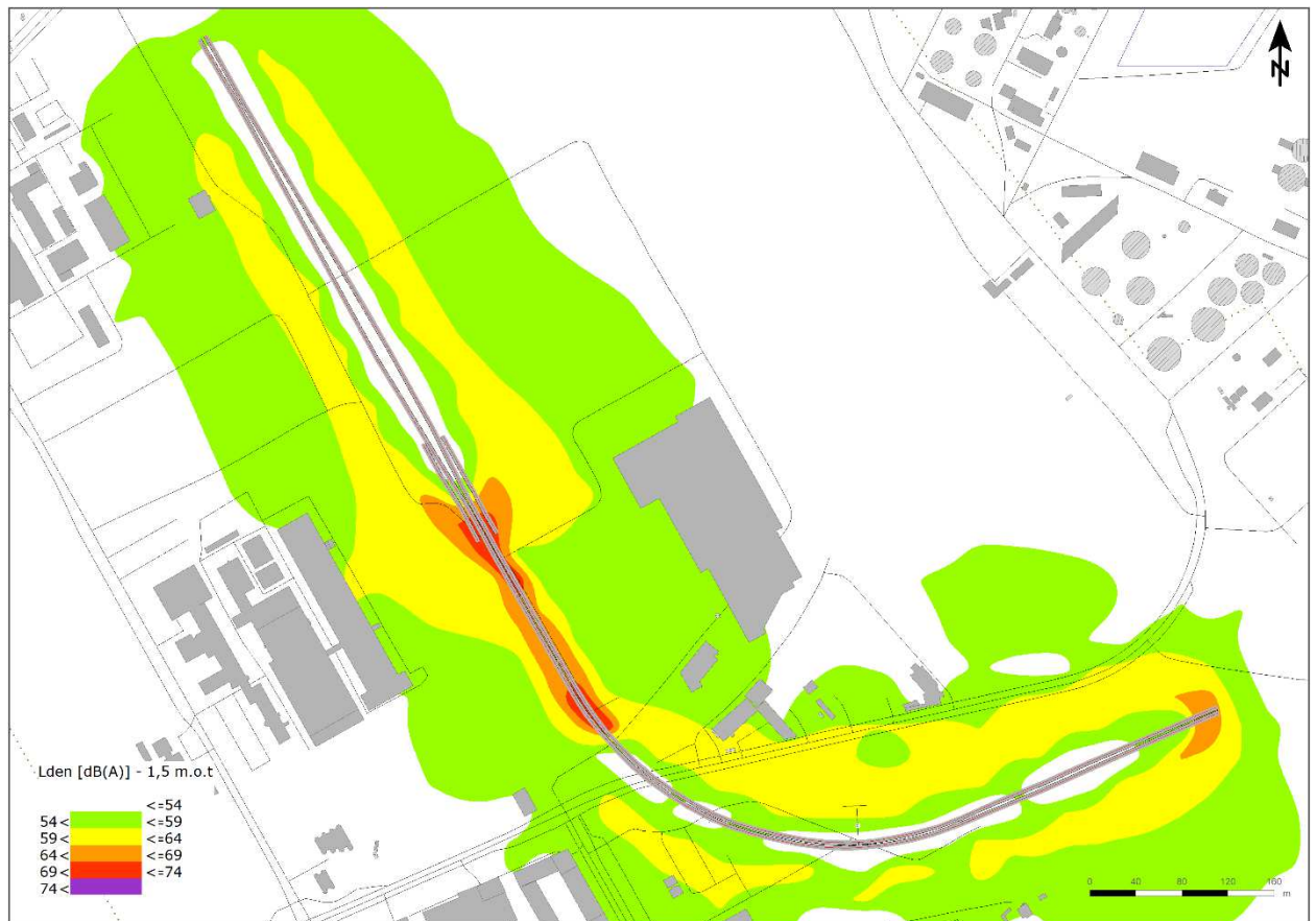
Figur 7-2 Støjudbredelse i 1,5 meter over terræn fra metrotrafik på M5's højbanestrækning uden integreret støjskærm på højbanen.
