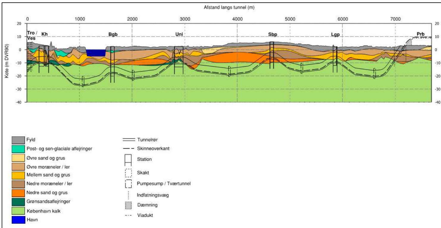
Figur 11-1 Geologisk profil fra Trommesalen (venstre) til Prags Boulevard (højre).
