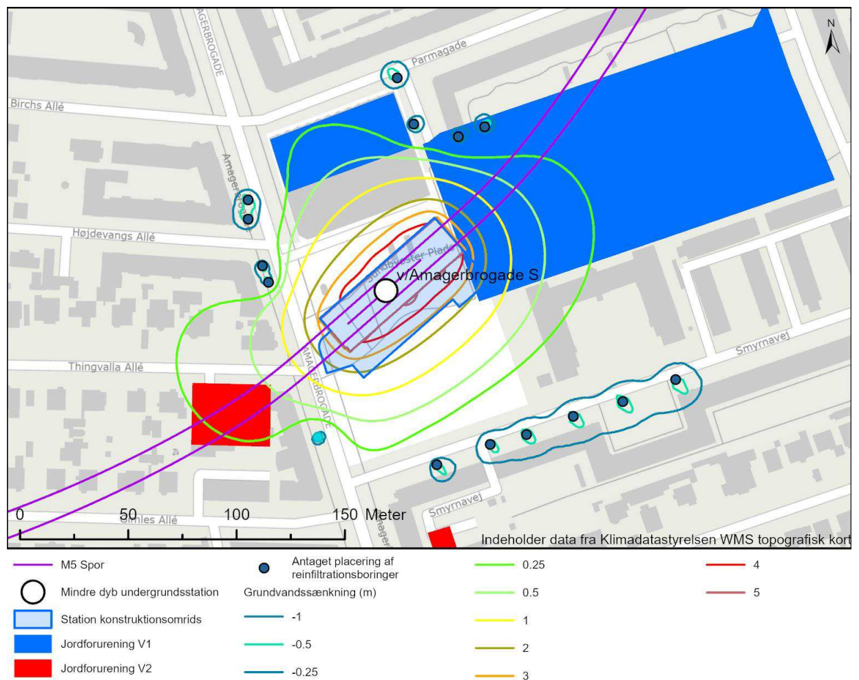
Figur 11-5 Beregnet sænkning i kalkmagasinet ved grundvandssænkning for v/ Amagerbrogade Syd med vægge til 5 m under bund udgravning og godt 90% reinfiltration.
