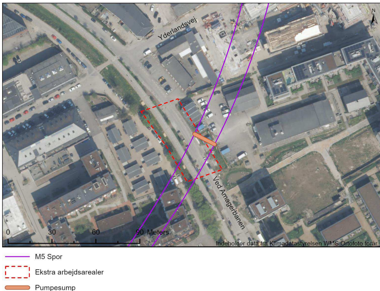
Figur 4-12 Placering af tværtunnel med pumpesump ved Amagerbanen.
