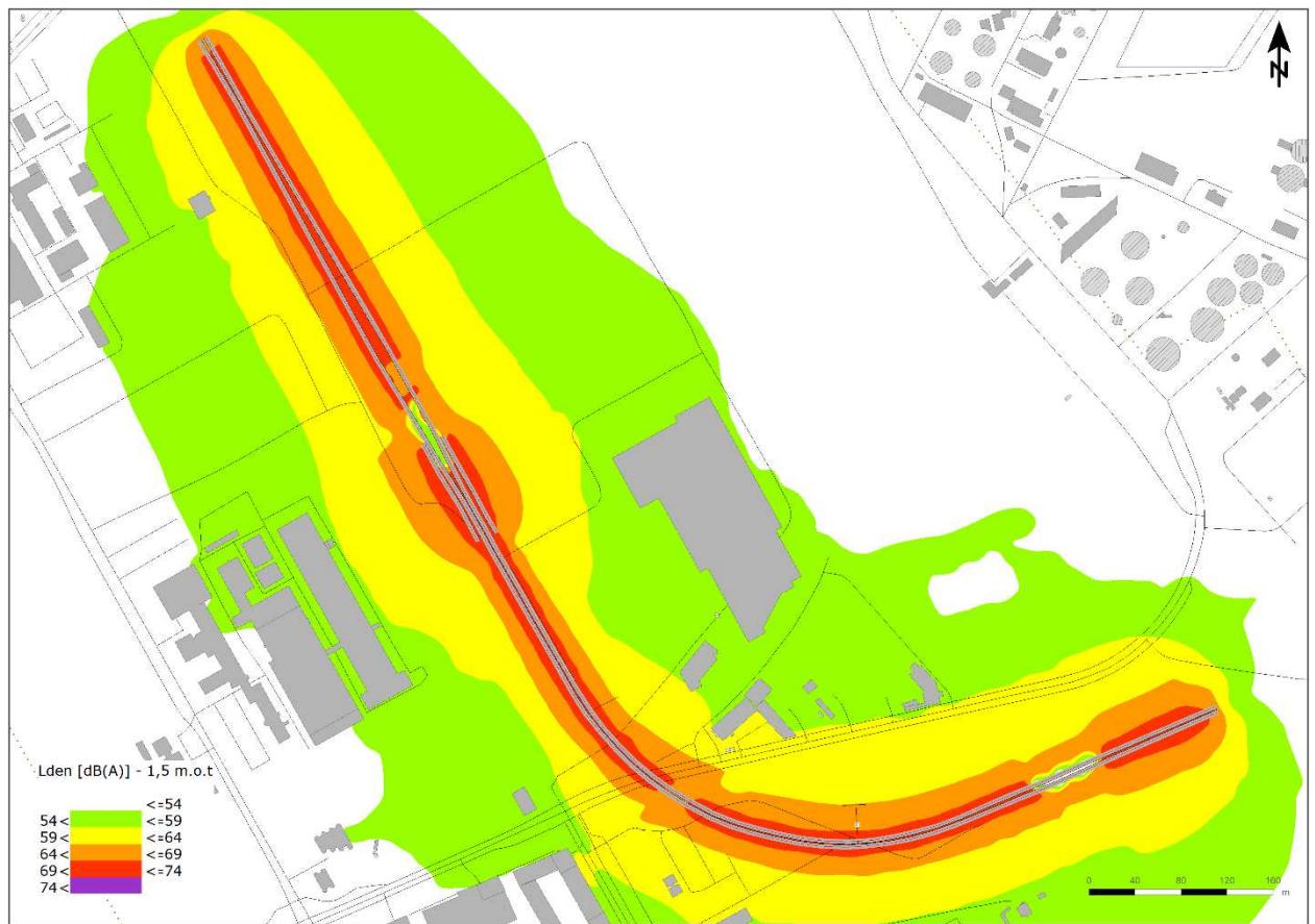
Figur 7-4 Støjudebredelse i 8 meter over terræn fra metrotrafik på M5 højbanestrækning uden integreret støjskærm på højbanen.
