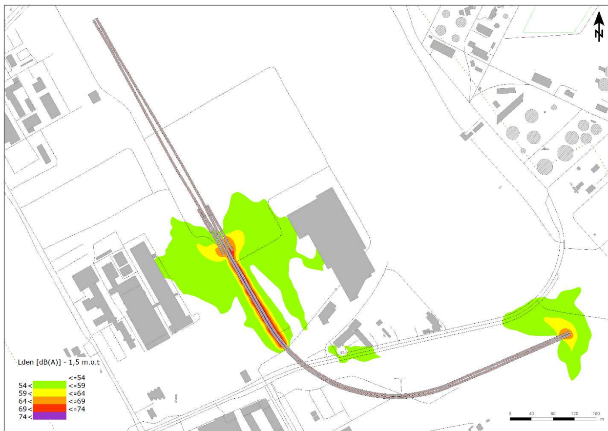
Figur 7-3 Støjudbredelse i 1,5 meter over terræn fra metrotrafik på M5's højbanestrækning inklusive en 0,6 meter høj støjskærm integreret på højbane.
