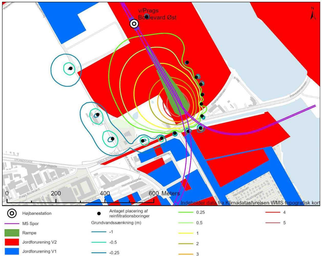
Figur 11-7 Beregnet sænkning i kalkmagasinet ved grundvandssænkning for rampe ved Prags Boulevard Øst med spunsvægge til kalkoverfladen, sekantpælevægge til 5 m under bund udgravning og ca. 98 % reinfiltration.
