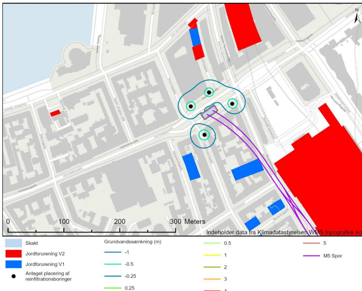
Figur 11-4 Beregnet sænkning i kalkmagasinet ved grundvandssænkning for skakt ved Vesterbrogade med vægge til 5 m under bund udgravning og knap 100% reinfiltration.
