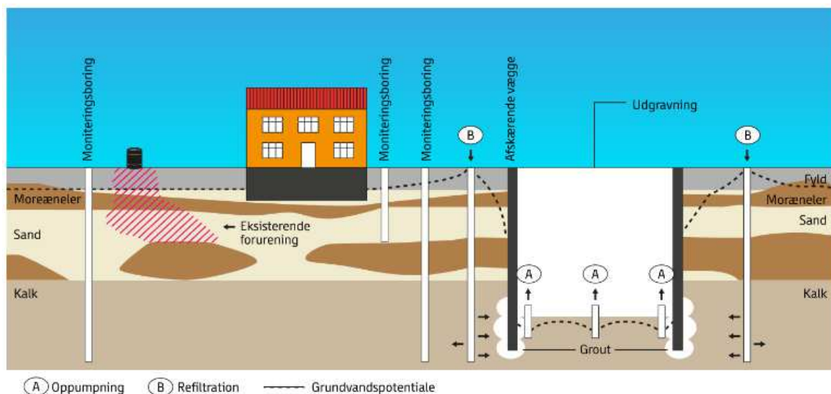
Figur 11-2 Princip for grundvandshåndtering.
