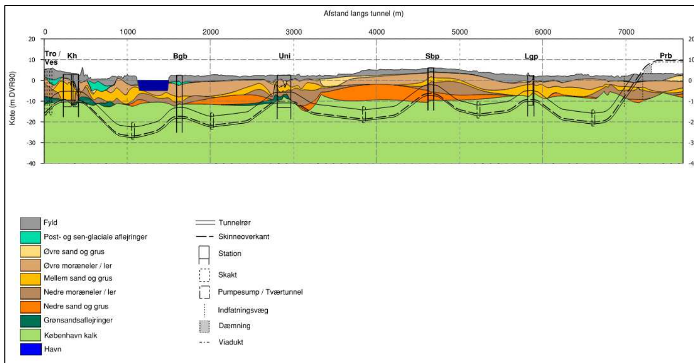
Figur 4-26 Opdateret længdeprofil mellem København H (Kh) og v/ Prags Boulevard Øst (Prb).
