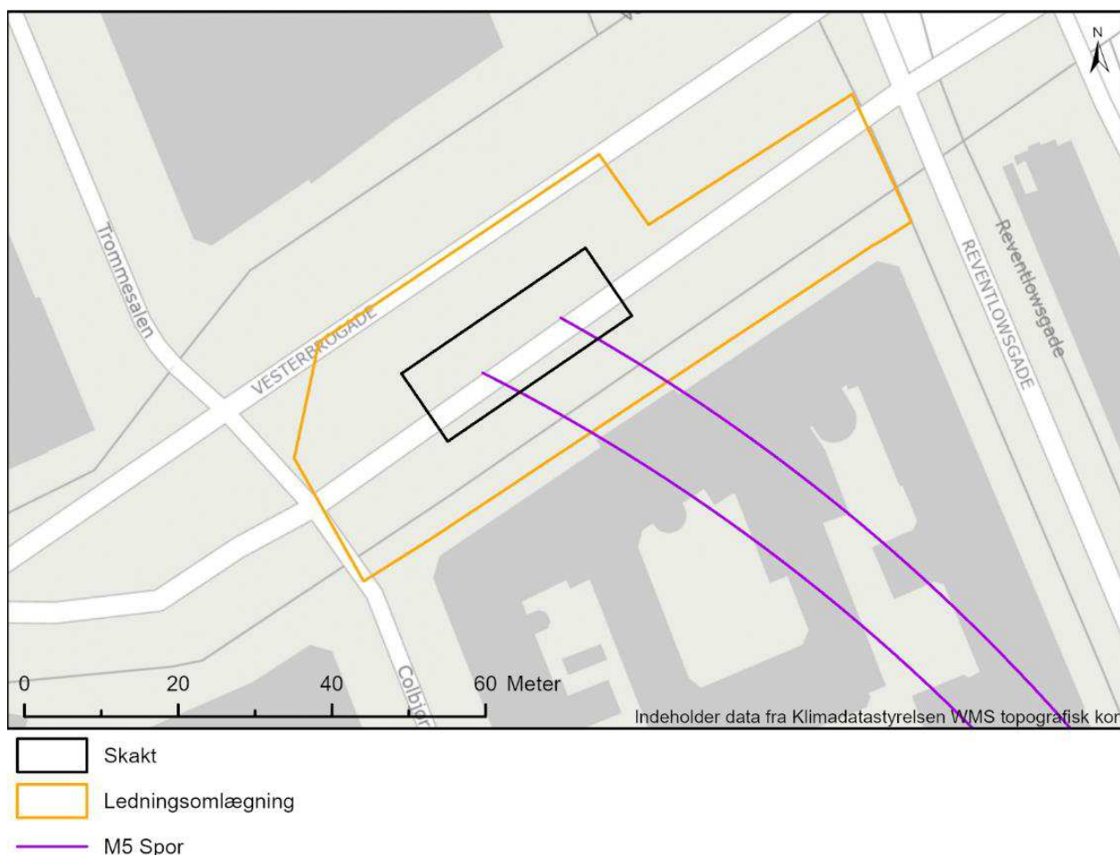
Figur 4-5 Arbejdsarealer til ledningsomlægninger ved Vesterbrogade.
