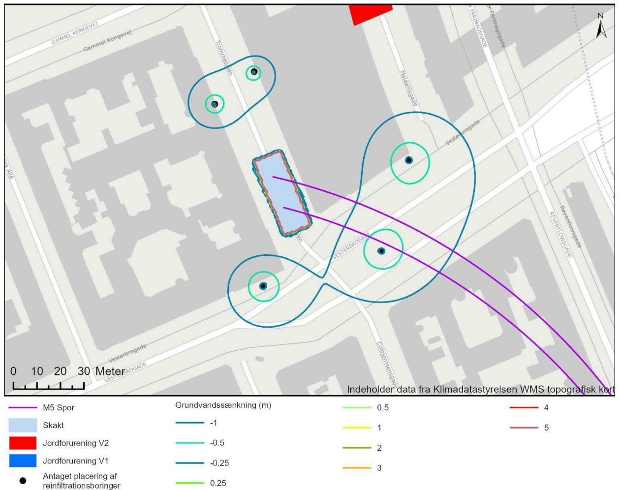
Figur 11-3 Beregnet sænkning i kalkmagasinet ved grundvandssænkning for skakt ved Trommesalen med vægge til 5 m under bund udgravning og ca. 90 % reinfiltration.
