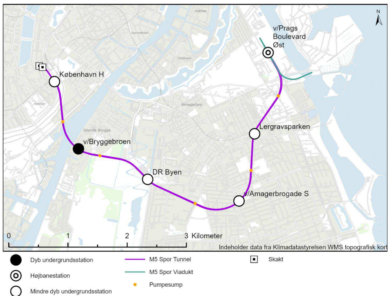
Figur 4-1 Oversigt over linjeføring med placering af stationer, skakte og tværtunneler med pumpeumpe, der indgår i denne supplerende MKV.
