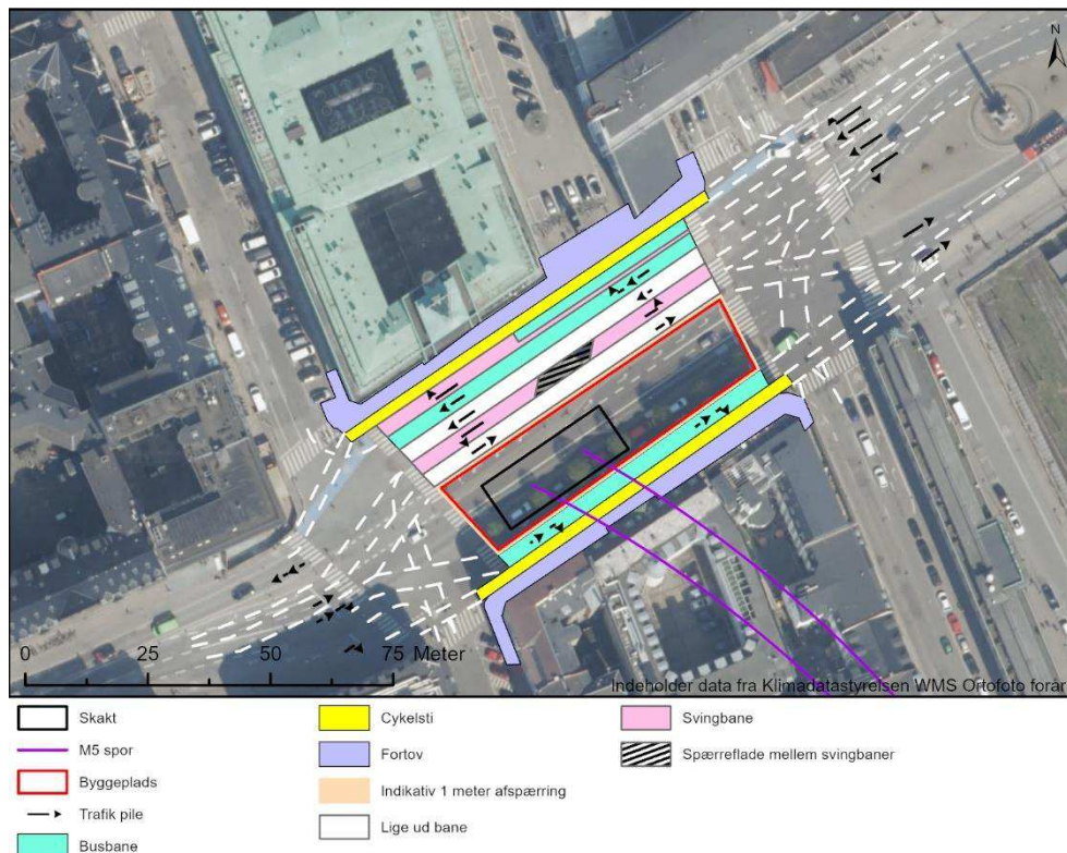
Figur 6-2 Forslag til trafikomlægninger på Vesterbrogade.
