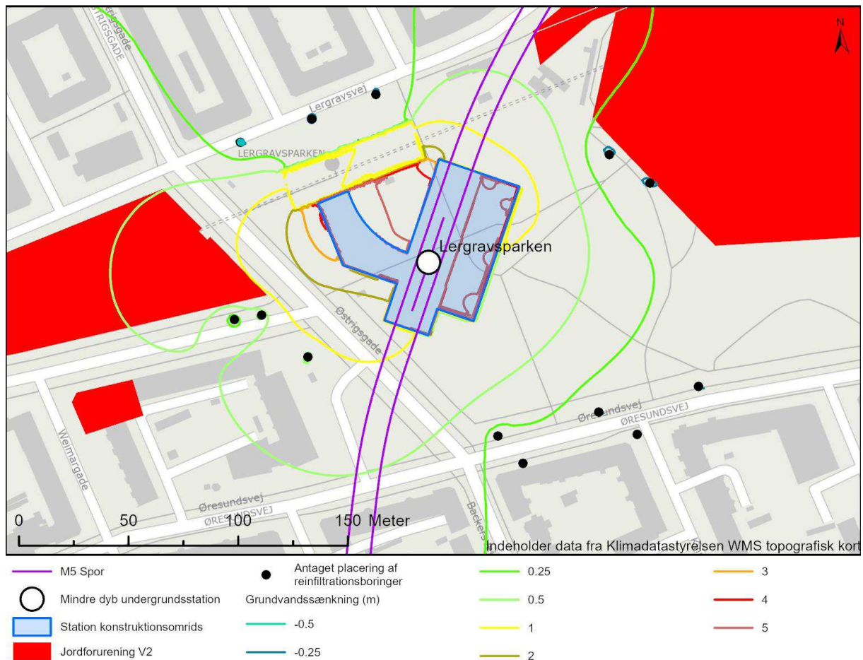
Figur 11-6 Beregnet sænkning i kalkmagasinet ved grundvandssænkning for Lergravsparken med vægge til 5 m under bund udgravning og knap 100% reinfiltration.
