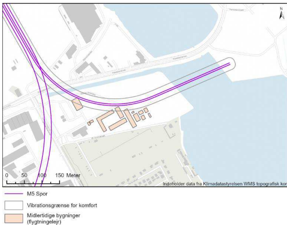
Figur 17-23 Vibrationskort for vibrationskomfort ved etablering af fundament til højbanestation ved Prags Boulevard (Prb).
