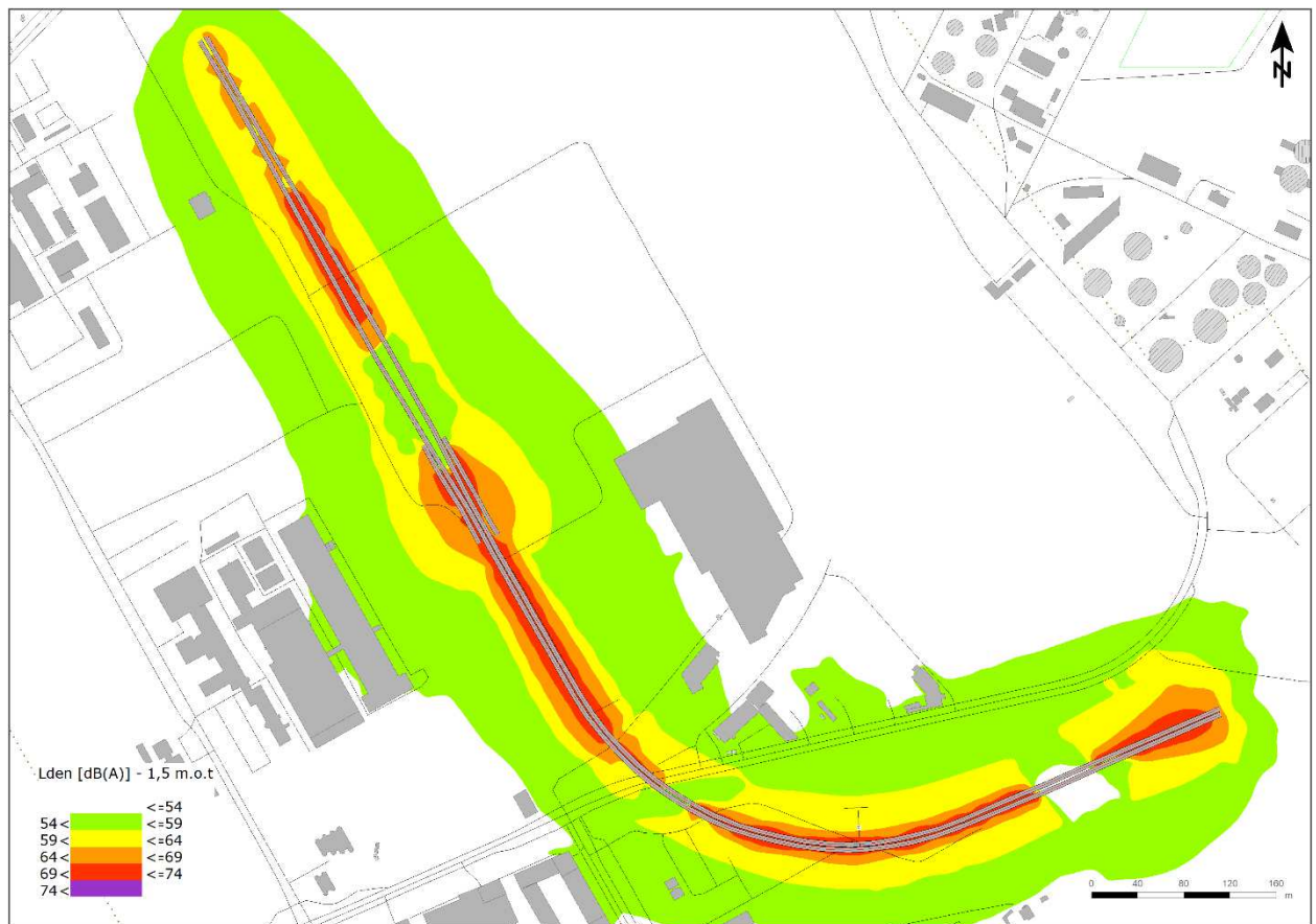
Figur 7-5 Støjudbredelse svarende til 3 etage (8 meter over terræn) fra metrotrafik på højbanestrækningen af M5 inklusive en 0,6 meter høj støjskærm integreret på højbane.
