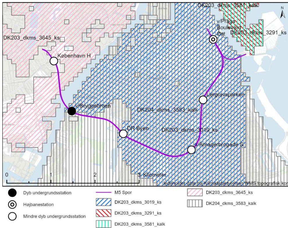
Figur 15-1 Placering af terrænnære grundvandsforekomster.
