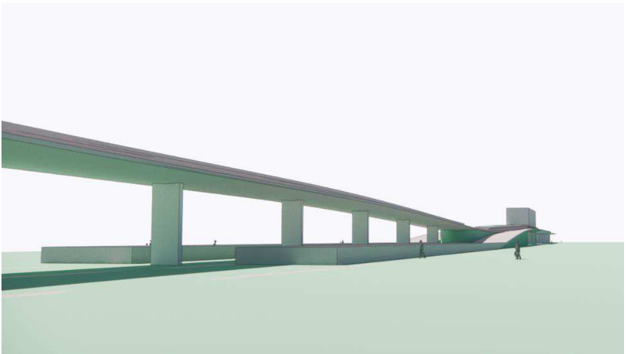
Figur 4-20 Skitse af viadukt til KVC, åben rampe og højbanestation ved v/ Prags Boulevard Øst set mod nord fra terræn.
