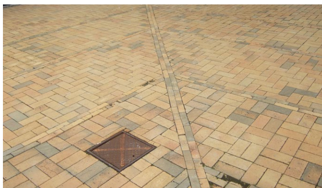
Sammenskæring og vandrende i teglbelægninger
