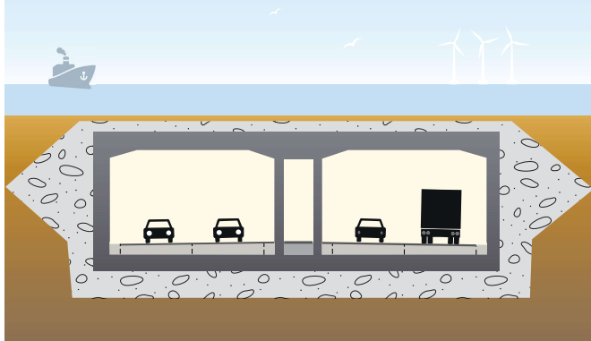
Figur 11: Sænketunnel.
