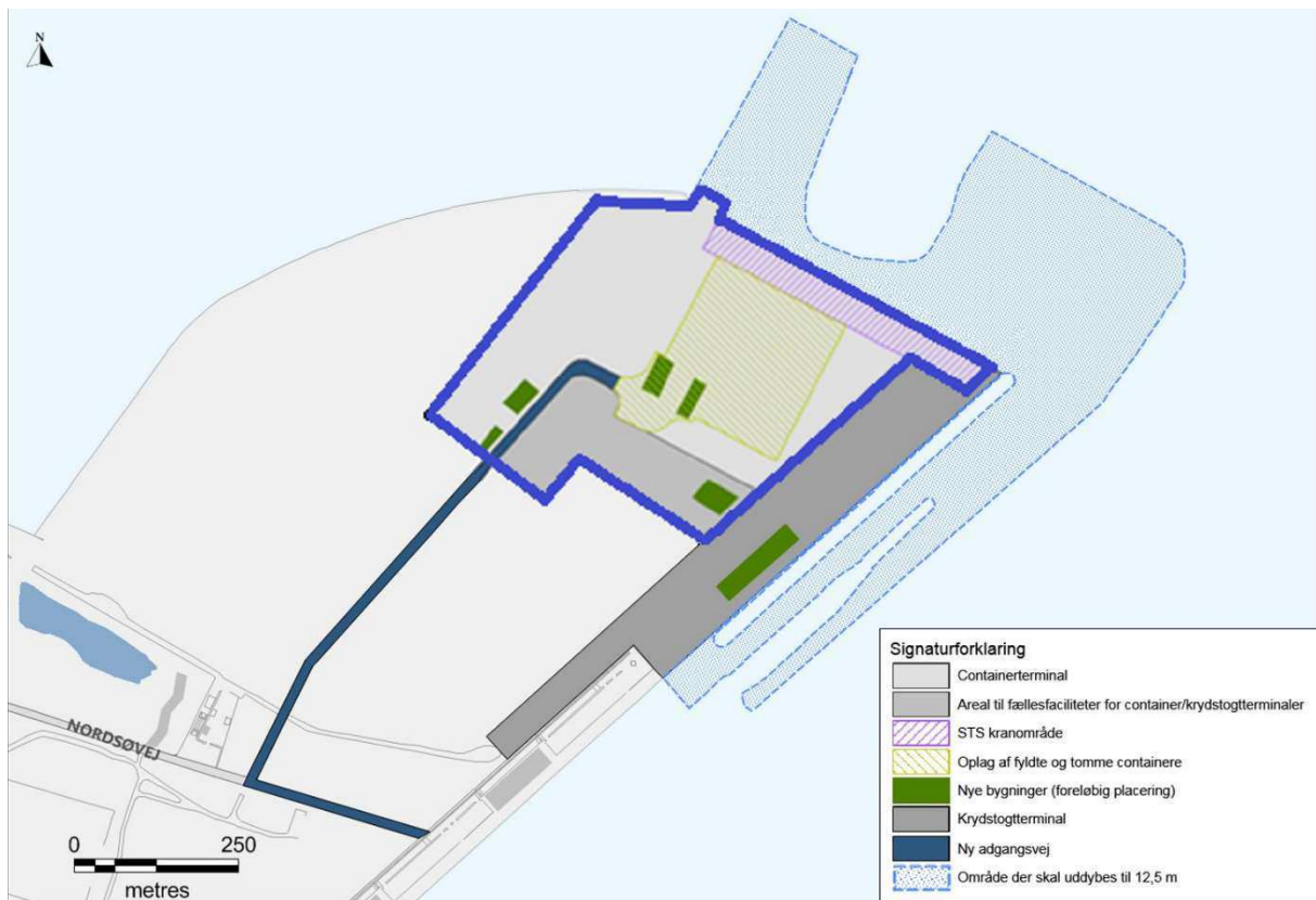
Figur D.2: Virksomhedens indretning. Den blå linje markerer projektgrænsen for nærværende ansøgning.
