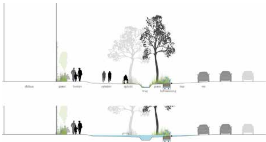
Udsnit ved Københavns Rådhus, øverst i tørvej, nederst ved skybrud. Bemærk, at der kun er vand på inderste vejbane.
