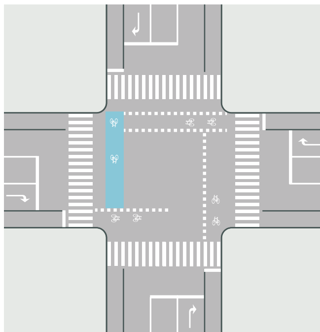
Figur 23: Kryds med kvart, halvt, helt og blåt cykelfelt
