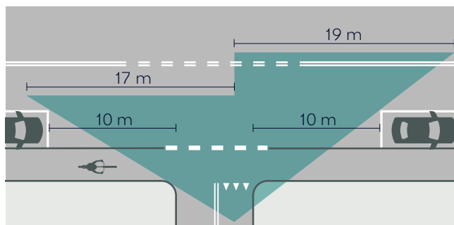
Figur 20: Oversigtsforhold med bilparkering 10 m fra sidevejen
