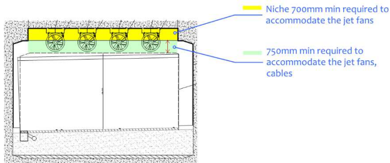
Figur 7-37 Ventilation-nicher til langsgående ventilation
