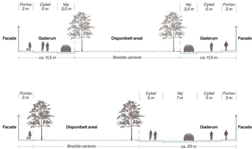
Figur 2-2 Principper for indretning af overfladearealet over tunnellerne. Arealet over tunnellerne kan designes og placeres på forskellige måder. Her er illustreret et princip, hvor det disponible areal kan ligge i midten i stil med en rambla eller i den ene side af byrummet, hvorved hele det disponible areal placeres tæt på den ene facade.
