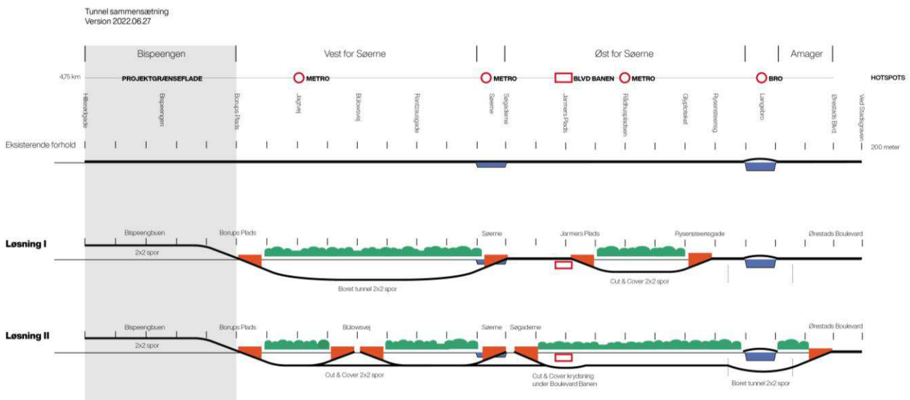
Figur 1-7 De to undersøgte løsninger i fase 1.
