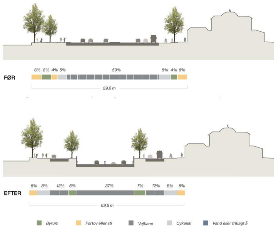
Figur 5-10 Eksempel på snit ved Søerne set mod vest
