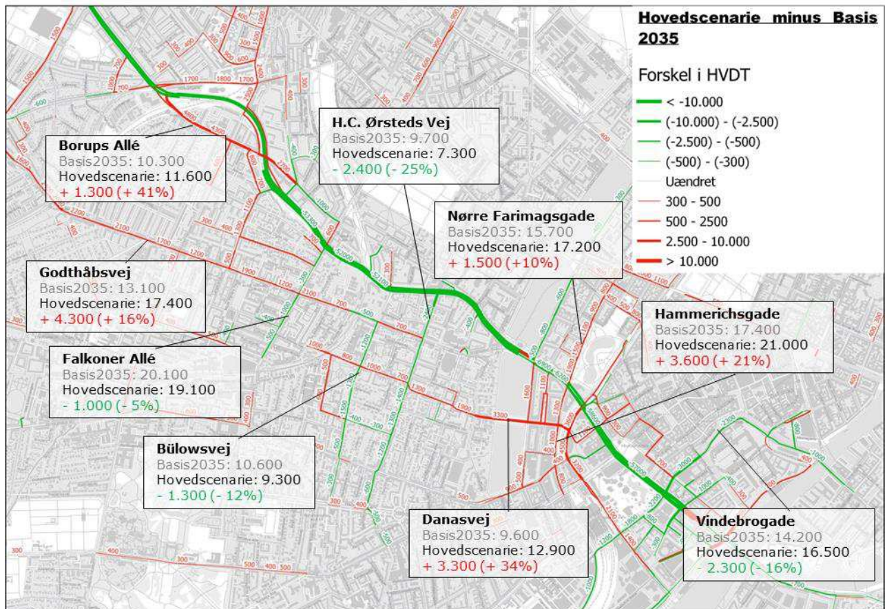
Figur 6-10 Illustration med fokus på trafikale ændringer på øvrige veje i Frederiksberg og København vist for gennemsnitlig hverdagsdøgtrafik (HVDT).
