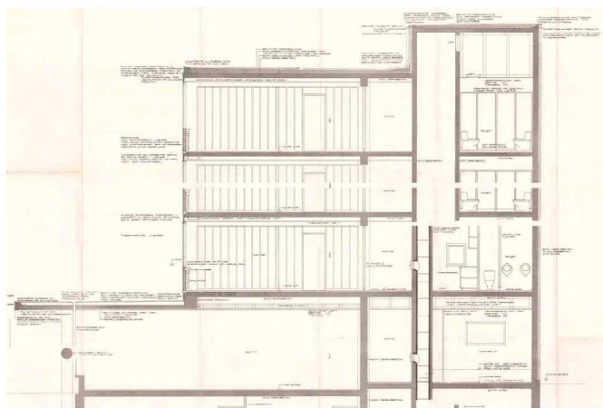
Illustration tværsnit i kontorbygningen fra 1961.
