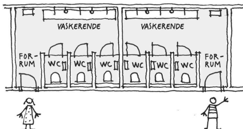
Skitse 2: Eksempel på disponering af kønsopdelte toiletter med vaskerende i forrum.
