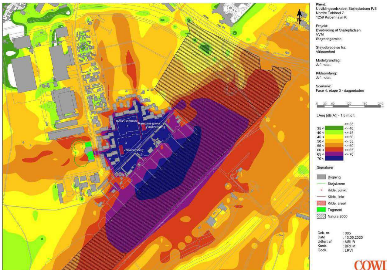
Figur 9-4 Støjkonturkort – fase 4 Pæleramning i byggezone J og G samt etablering af kældere ved spunsning i byggezone F.
