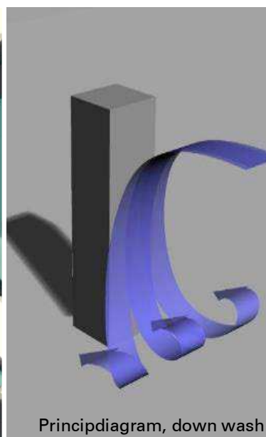
Figur 9 Strømlinjer viser, hvordan vinden kommer ind på den østlige plads. For vind fra SØ og vest. Samt principdiagram for down wash.
