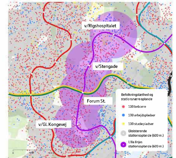
Figur 2: Linjeføring og stationsnærhed for perspektivstrækningen på M5 mellem København H og Østerport (varianten inkl. station ved GL Kongevej)
