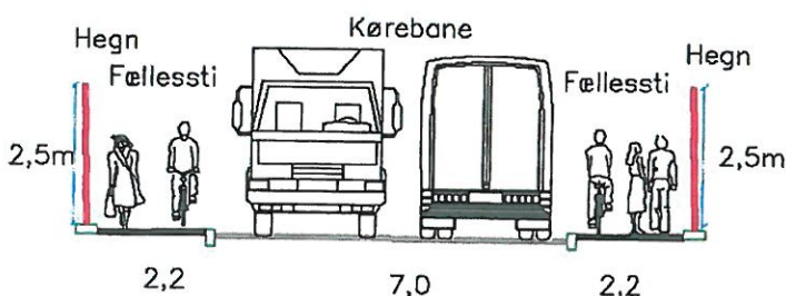
Figur 2. Tværsnit af nyt vejprofil syd for Sundkrogsgade.
