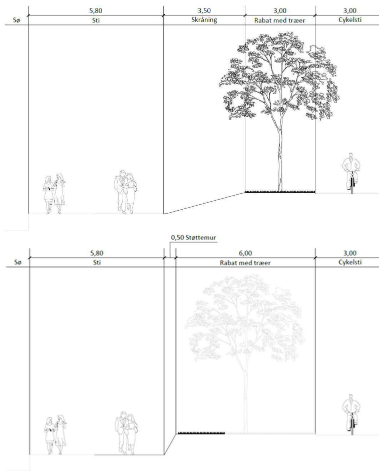
Figur 31: Øverst: Eksisterende tværsnit. Midten: fremtidigt tværsnit, hvis skrænten flyttes tre meter længere væk fra søen og træerne genplantes. Nederst: Fremtidigt tværsnit, hvis skrænten erstattes af en støttemur og træerne bevares.
