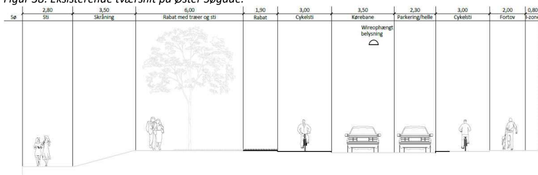
Figur 39: Fremtidigt tværsnit i løsningsforslag 01.
