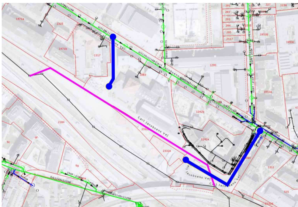
Figur 4 – HOFOR tilslutningsmuligheder for projektområdet
