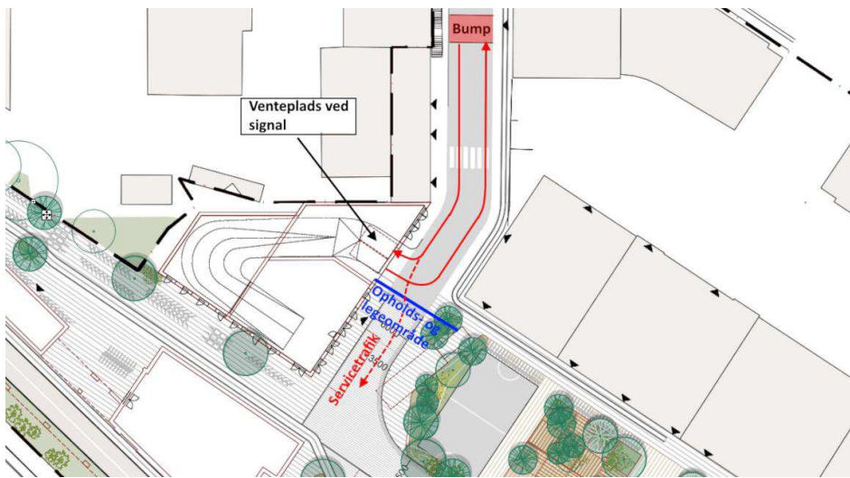
Figur 5-1: Trafikal løsning ved parkeringsrampen, med indsnævring til ét kørespor.
