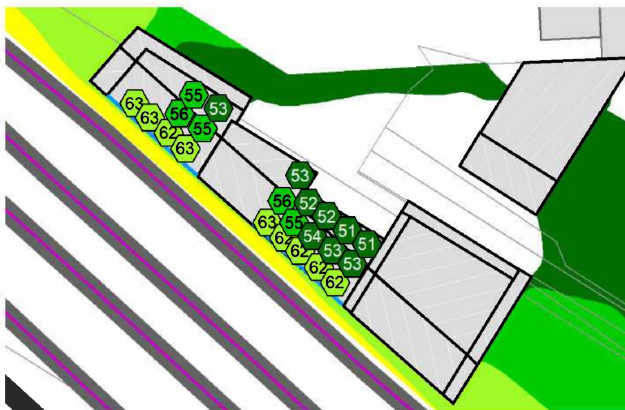
Figur 10b: Beregnet jernbanestøjbelastning L_{den} i dB på tagterrasse af BF3.
