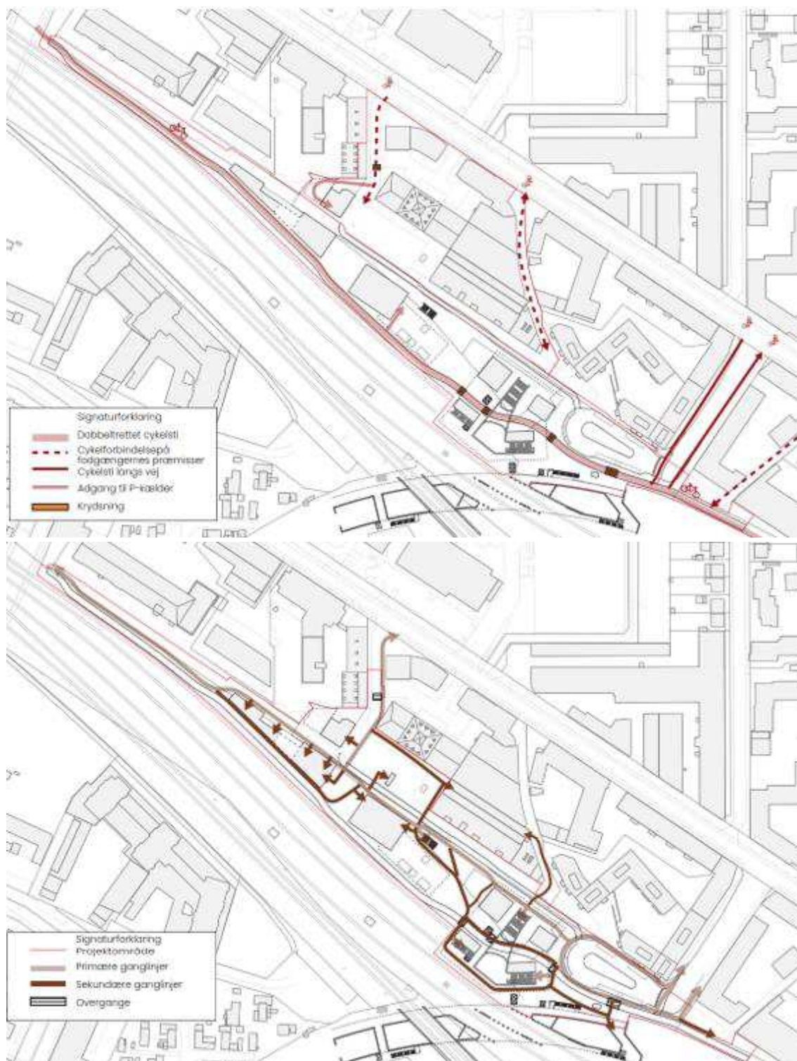
Figur 10.3: Planlagte forhold for cyklister i planområdet /bilag 4/.
