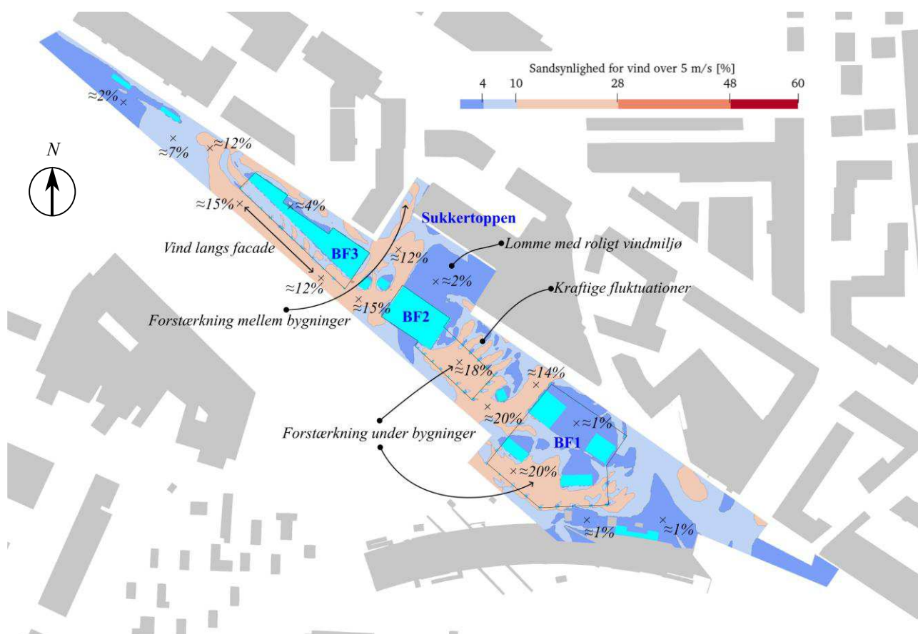
Figur 5. Sandsynlighed for at vindhastigheden overskrider 5 m/s i terrænniveau i området omkring projekt København Syd By. Niveaufladerne er farvet efter de øvre grænseværdier for 'acceptabelt' for de forskellige aktivitetskategorier i Tabel 1. Der er i udvalgte punkter angivet den numeriske værdi af den beregnede overskridelsessandsynlighed.
