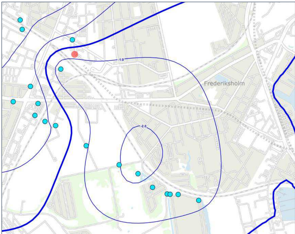
Figur 1.3 Grundvandspotentialet i det primære kalkmagasin. Byggefeltet er markeret med rød prik. Bemærk grundvandssænkningen til ca. -2,0 mDVR90 SØ for byggefeltet.
