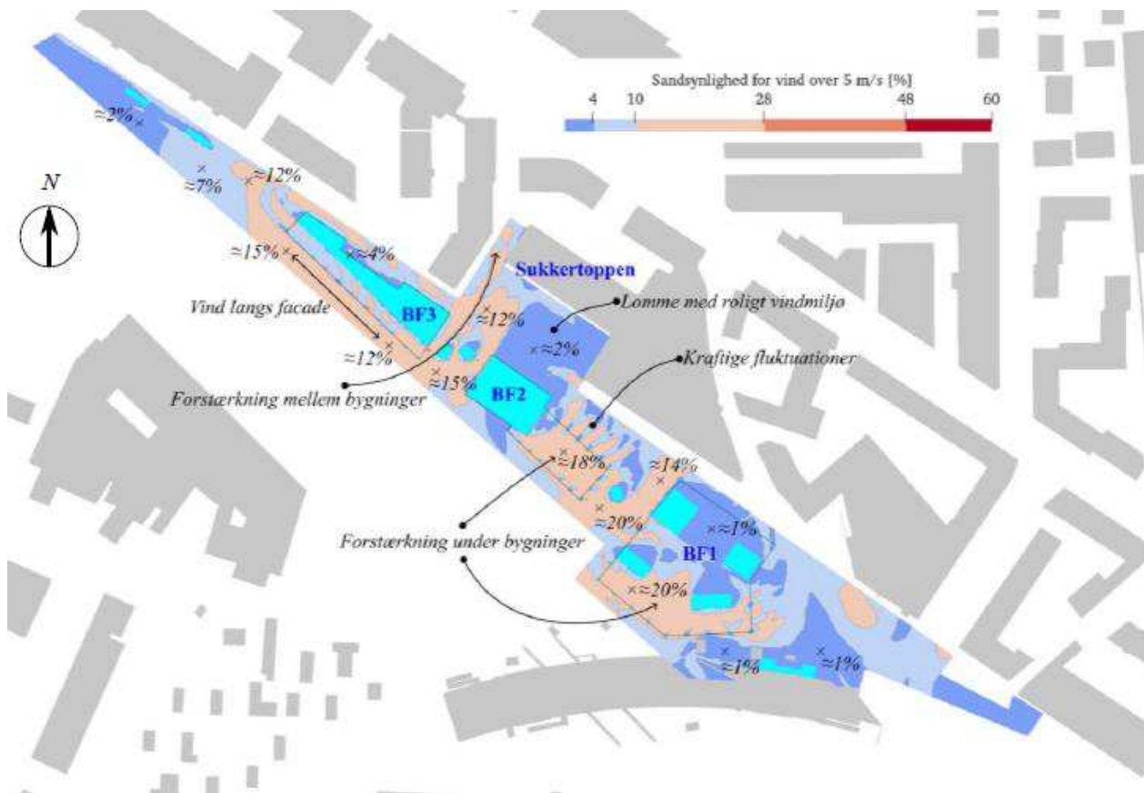
Figur 9.5: Oversigtskort over den beregnede sandsynlighed for, at vindhastigheder overskrider 5 m/s i området omkring planområdet. Den numeriske værdi af den beregnede overskridelsessandsynlighed er angivet i udvalgte punkter /bilag 1/.
