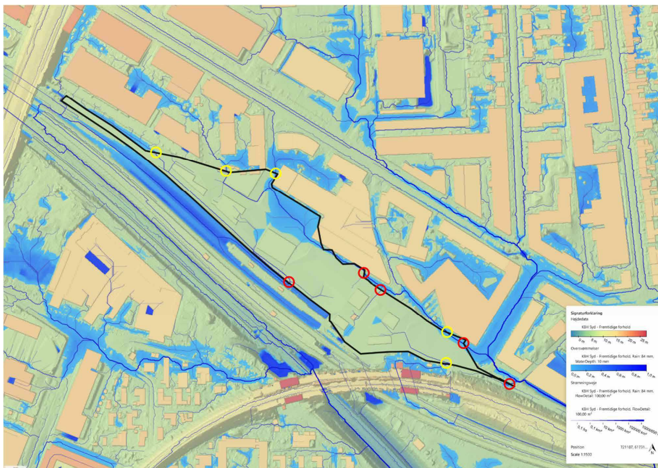
Figur 13 – Scalgoanalyse ekstremregn, strømningsveje fremtidige forhold
