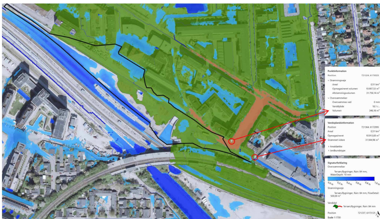
Figur 22 – Vandomland nord, eksisterende forhold
