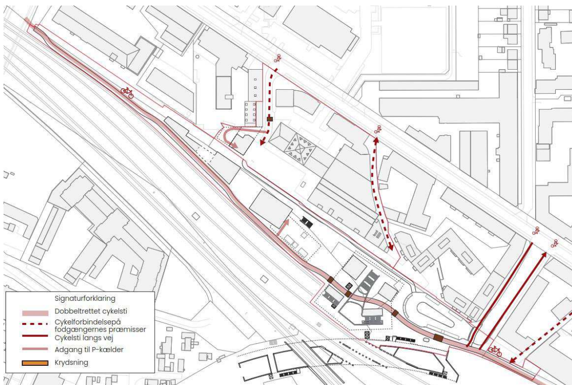
Figur 4-1: Planlagte cykelforhold i projektområdet (illustration fra Byrumskatalog)
