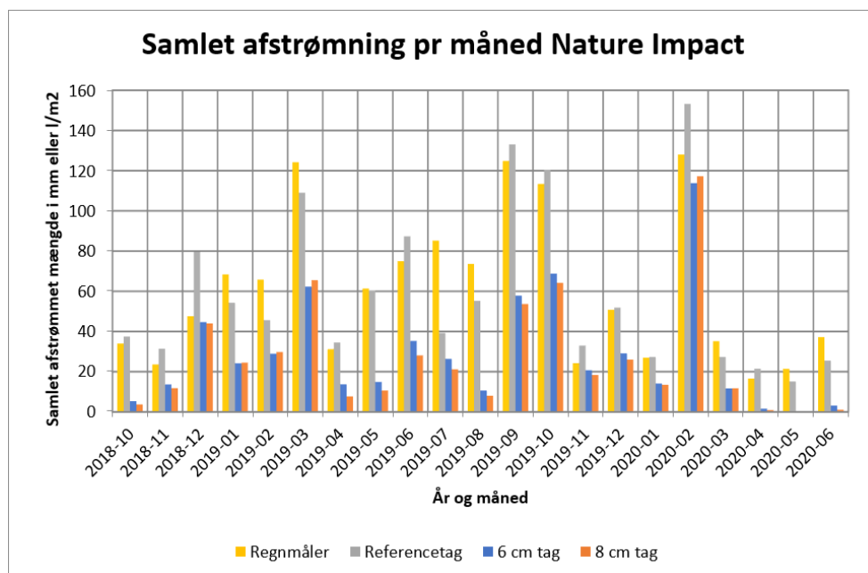
Figur 3-8 Samlet afstrømning pr. måned i forhold til den samlede nedbør pr. måned.
