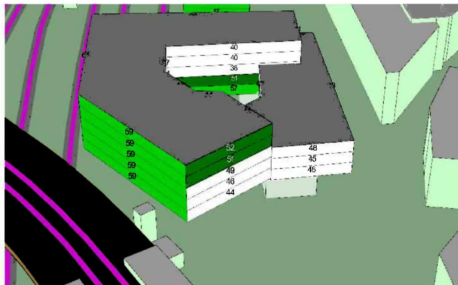
Figur 3: Beregnet jernbanestøj L_{den} i dB, Byggefelt 1 (kontor), set fra syd.
