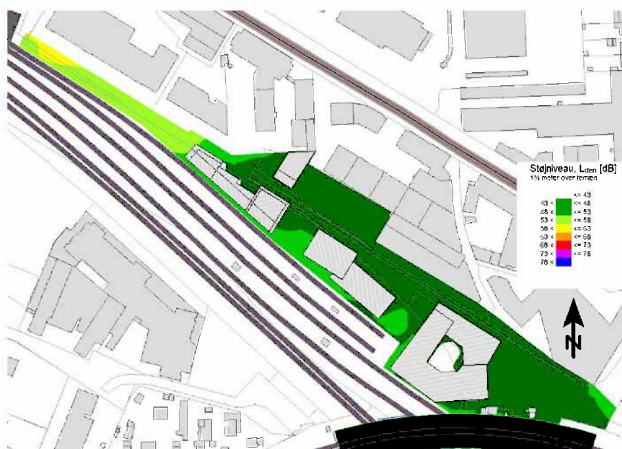
Figur 17: Beregnet vejstøjbelastning L_{den} i dB på planområdets udearealer.
