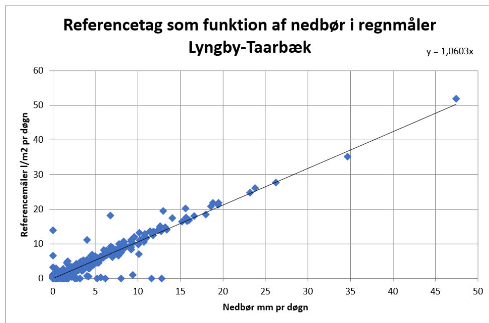
Figur 3-1 Døgnværdier af afstrømningen fra referencetaget som funktion af døgn-nedbørsværdien.
