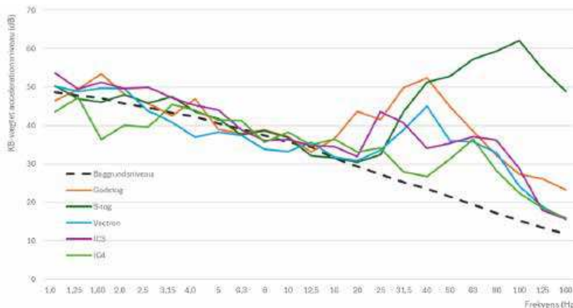
Figur 9.31: De typiske KB-vægtede maksimalværdier for de registrerede togpassagerer for de forskellige togtyper pr. 1/3-oktavbånd /bilag 3/.
