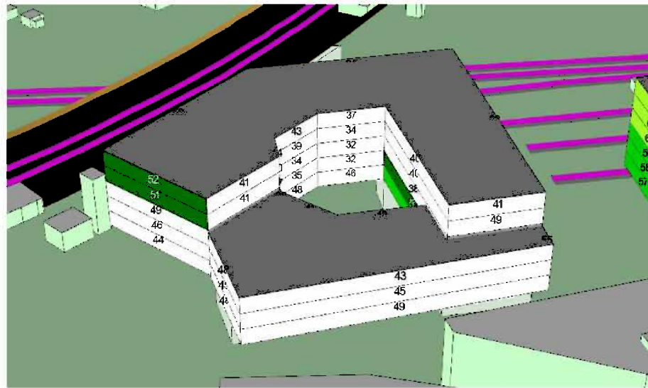
Figur 4: Beregnet jernbanestøj L_{den} i dB, Byggefelt 1 (kontor), set fra øst.
