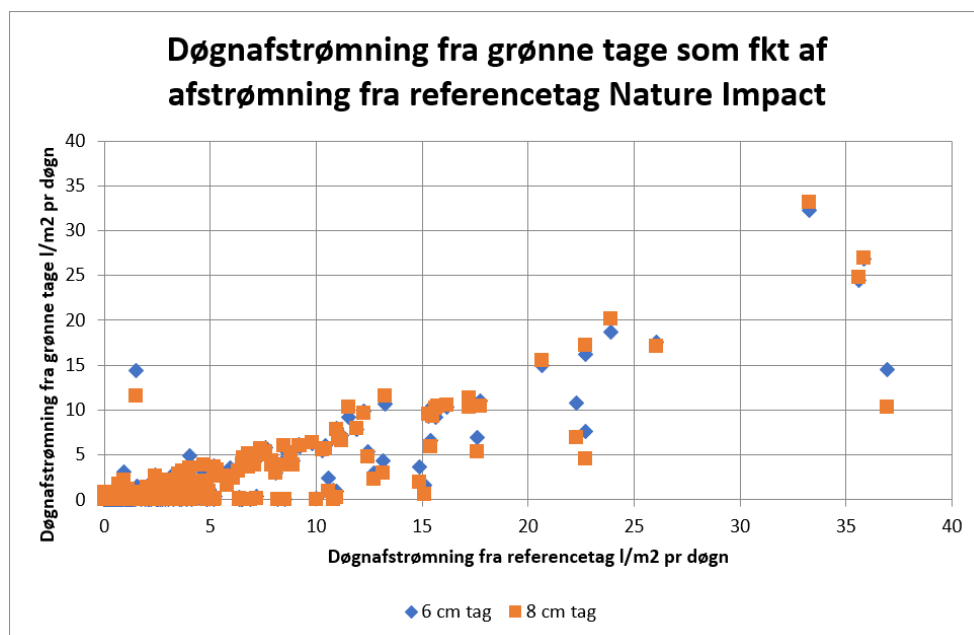
Figur 3-6 Døgnafstrømningen fra de grønne tage hos Nature Impact som funktion af døgnafstrømningen fra referencetaget.
