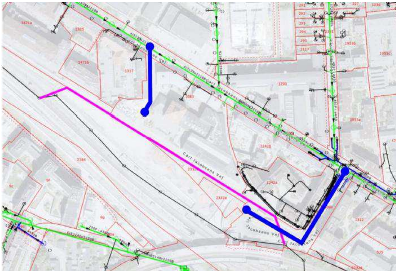
Figur 12.5: Kommende tilslutninger for planområdet /Bilag 6/.
