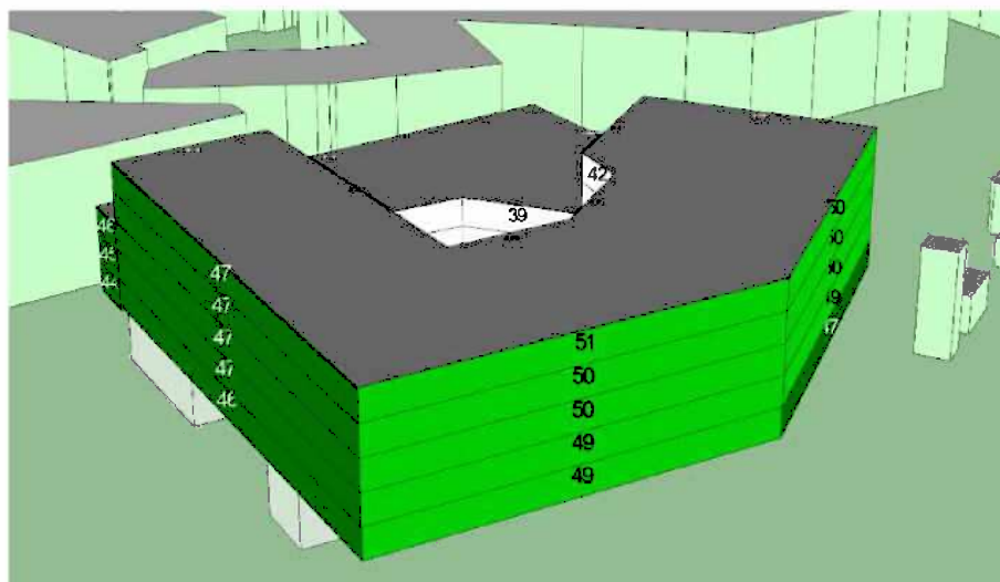
Figur 11: Beregnet vejstøjbelastning L_{den} i dB, Byggefelt 1, set fra vest.
