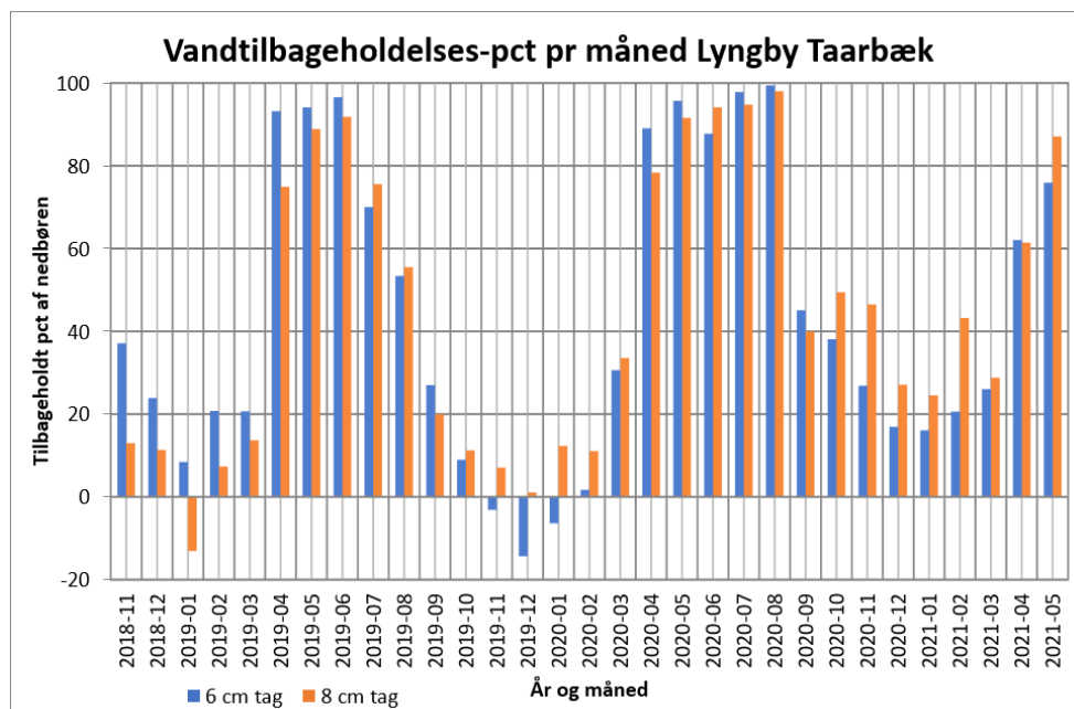
Figur 3-3 Vandtilbageholdelsesprocenten på månedsbasis for de to grønne tage.
