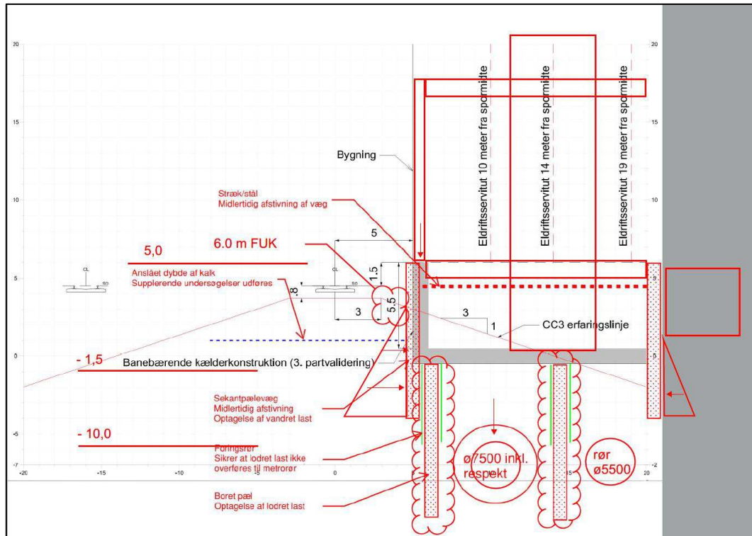
Figur 1.6: BF3, skitsetværsnit fremsendt af Ingcon. Udgravningsniveauet er efterfølgende ændret til kote -0,5.
