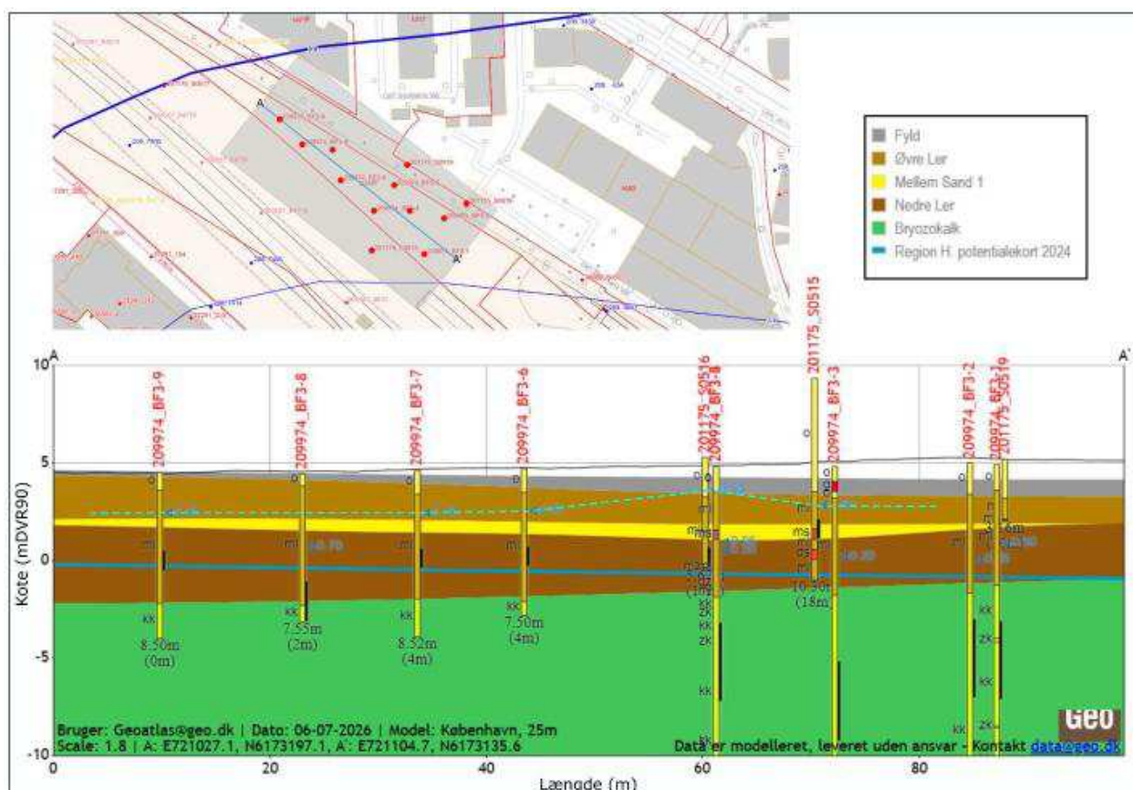
Figur 12.10: Geologisk profil med boringer og pejlinger. Det terrænnære grundvandsspejl er markeret med turkis stiplede linje. Det forventede potentiale for det primære grundvandsspejl er angivet med blå linje/Bilag 7/.
