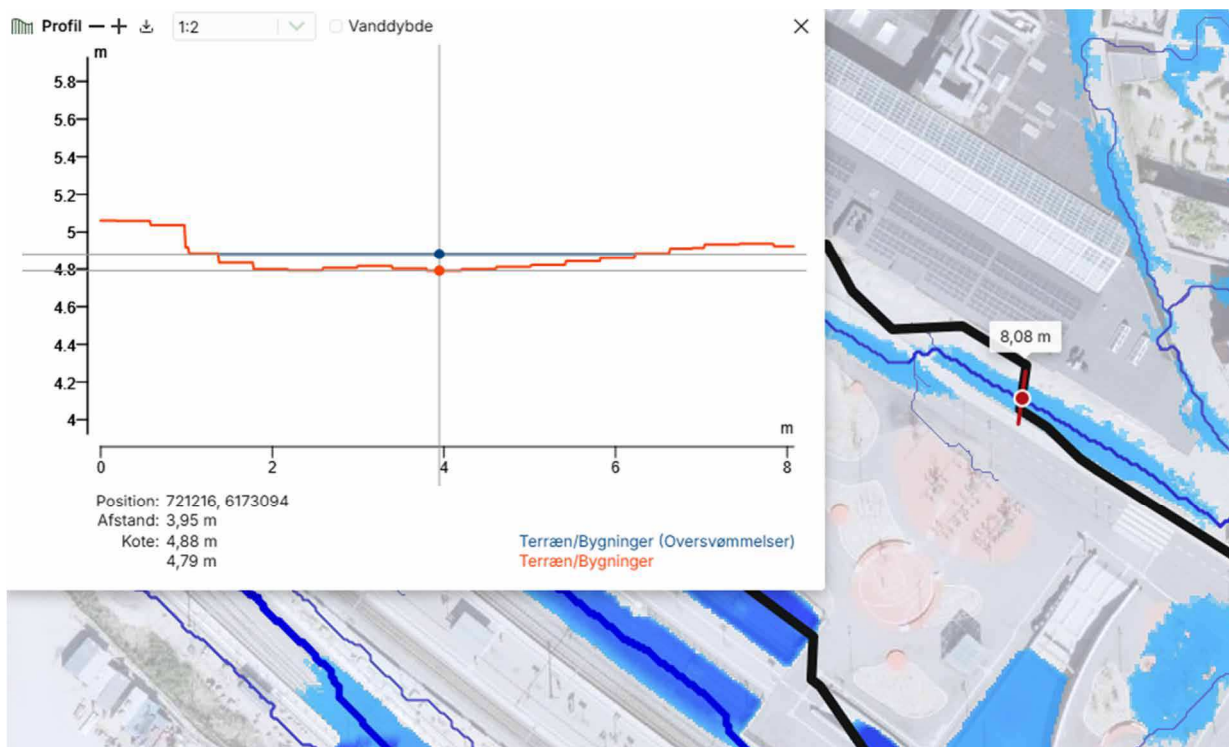
Figur 9 – Kote for afstrømning ud af området
