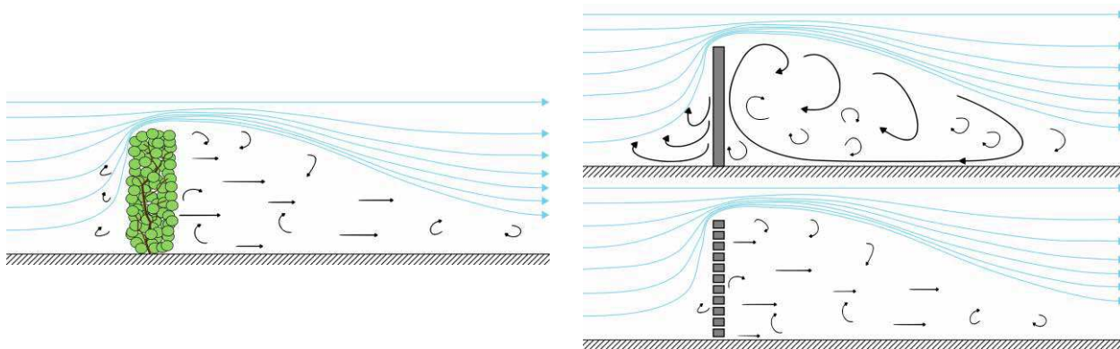
Figur 6. Lægivere: Bevoksning (til venstre) giver pga. dens gennemtrængelighed godt læ ved at reducere store hvirveldannelser. Tætte læskærme (øverst til højre) kan medføre risiko for kraftig turbulens bag skærmene, mens åbninger i skærmene (nederst til højre) reducerer denne.
