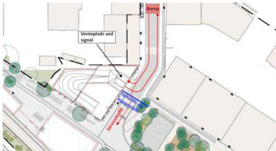
Figur 10.5: Trafikløsning ved rampen til parkeringskælderen /Bilag 4/.
