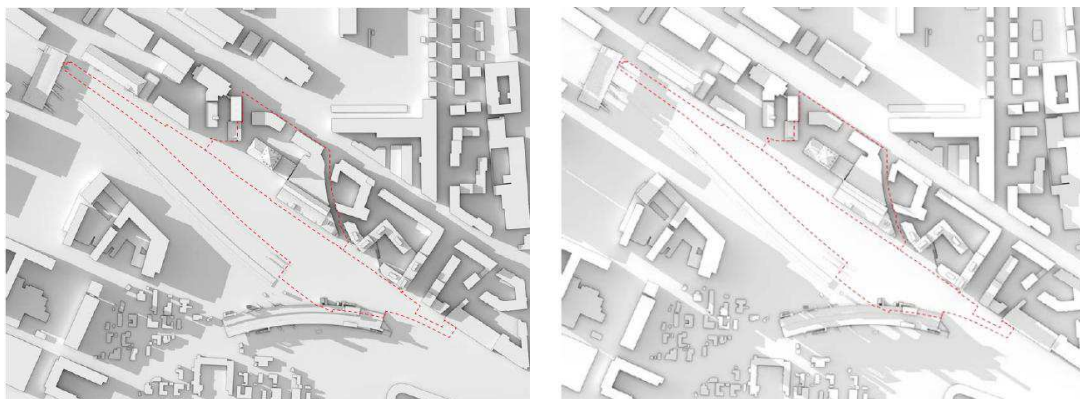
Figur 9.12: Skyggediagrammer for de eksisterende forhold ved sommarsolhverv, d. 21. juni. Tv.: Kl. 20.00. Th.: Kl. 21.00. Planområdet er markeret med rød.
