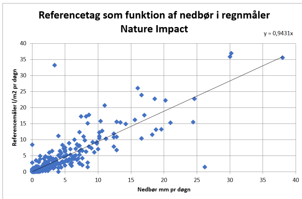
Figur 3-5 Døgnafstrømning fra referencetaget hos Nature Impact som funktion af døgnnedbøren.
