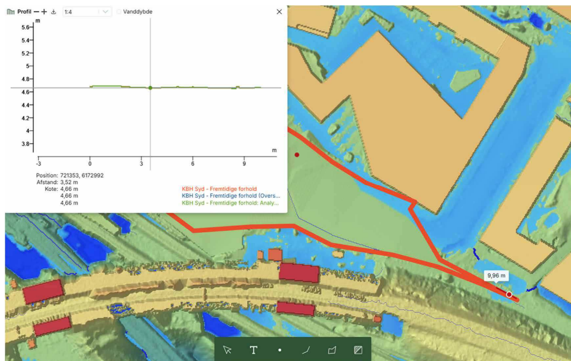
Figur 15 – Kote for afstrømning ud af området
