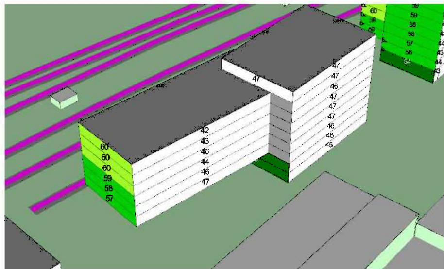
Figur 6: Beregnet jernbanestøj L_{den} i dB, Byggefelt 2 (hotel), set fra øst.
