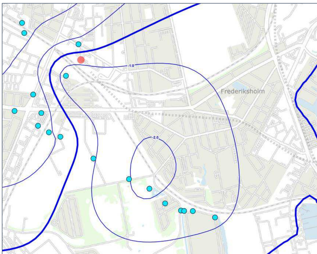
Figur 2 Grundvandspotentialet i det primære kalkmagasin. Byggefeltet er markeret med rød prik. Bemærk grundvandssænkningen til ca. -2,0 mDVR90 SØ for byggefeltet.
