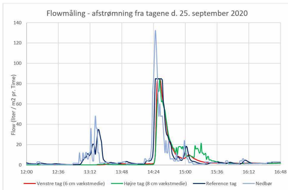
Figur 4-3 Forstørret billede af nedbørsintensiteten og afstrømningen under selve skybruddet. De lidt underlige stigninger i afstrømningen efter kl. 15 fra det højre tag er der ikke umiddelbart en forklaring på.
