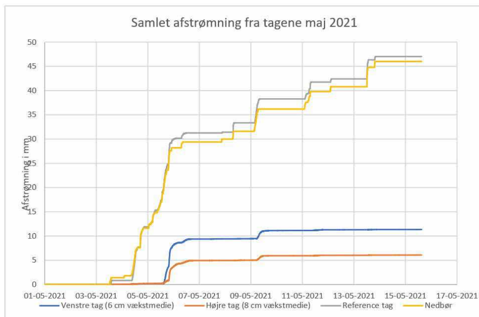
Figur 6-1 Summeret afstrømning og nedbør i maj måned 2021.
