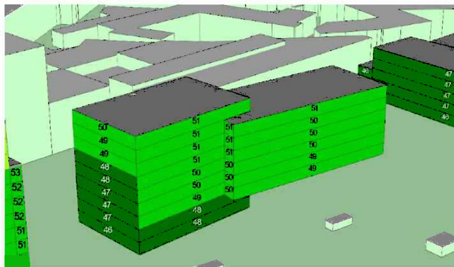
Figur 13: Beregnet vejstøjbelastning L_{den} i dB, Byggefelt 2, set fra vest.
