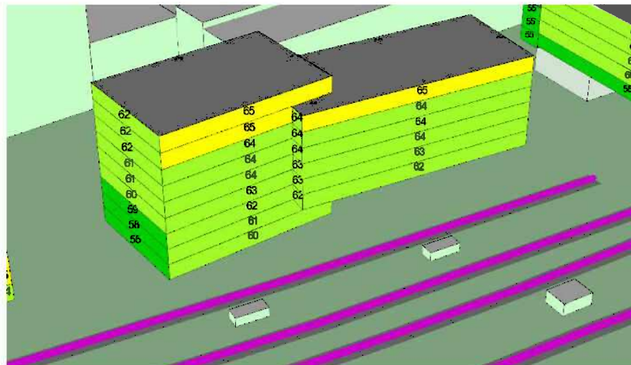
Figur 5: Beregnet jernbanestøj L_{den} i dB bebyggelsen, Byggefelt 2 (hotel), set fra vest.
