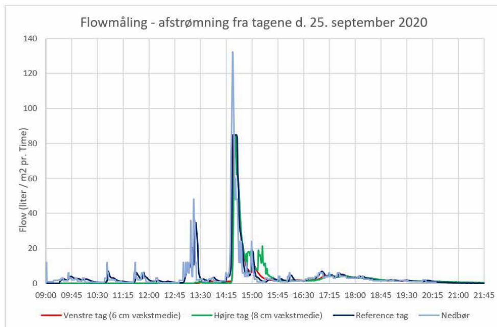
Figur 4-2 Flow fra de tre tage i l/m 2 pr. time sammenlignet med regnintensiteten målt i mm pr. time med SVK5628 regnmåleren, som fysisk står lige ved siden af de grønne tage.
