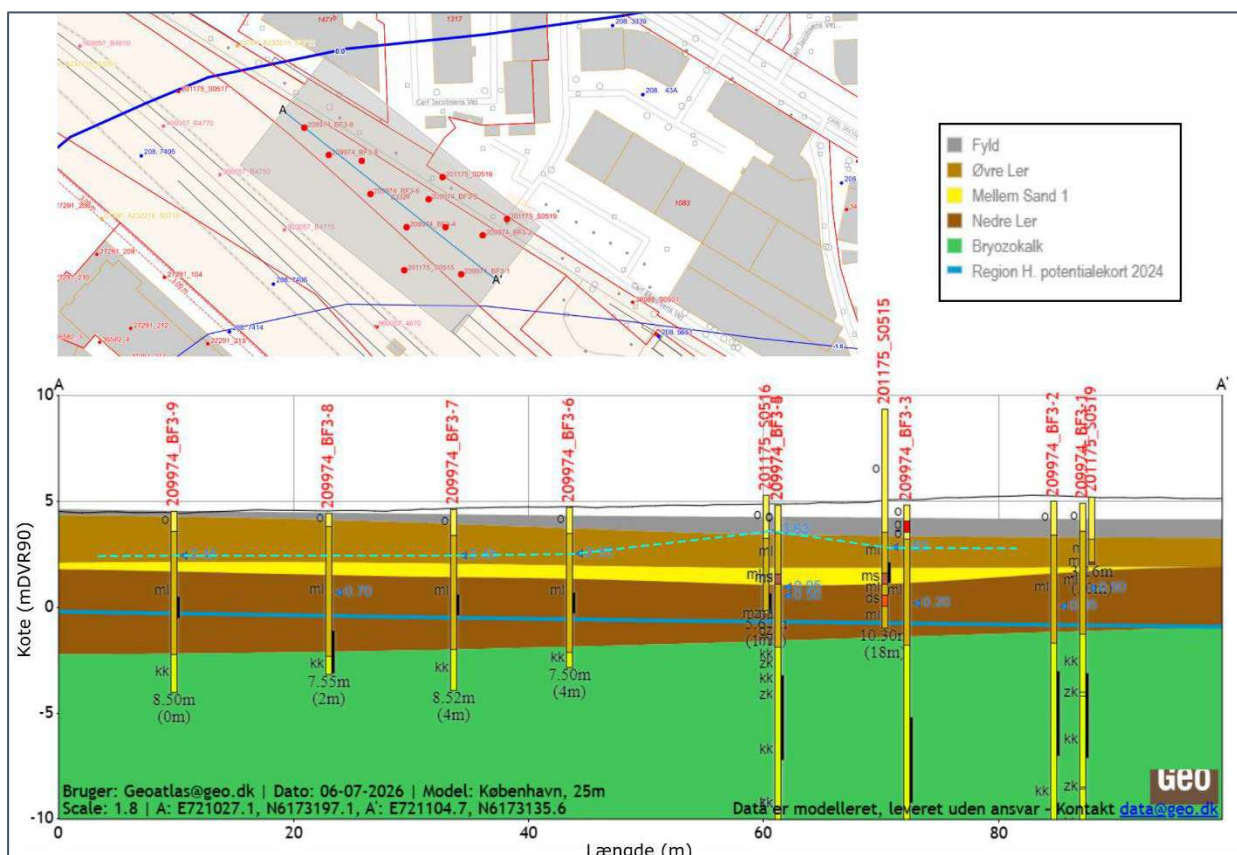
Figur 1 Geologisk profil fra GeoAtlas Live med boringer og pejlinger vist. Det terrænnære grundvandspejl er markeret med turkis stiplede linje. Det forventede potentiale for det primære grundvandspejl er vist med blå linje.
