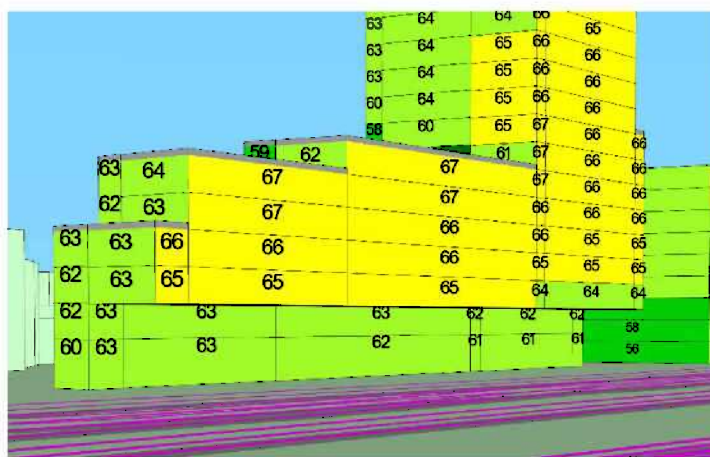
Figur 9: Beregnet jernbanestøj L_{den} i dB, Byggefelt 3 (bolig), set fra vest, stueetagen.
