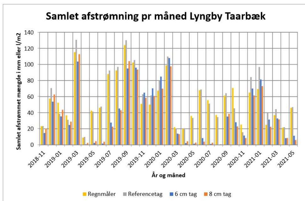
Figur 3-4 Samlet afstrømning pr. måned fra de tre tage samt samlet nedbør pr. måned.
