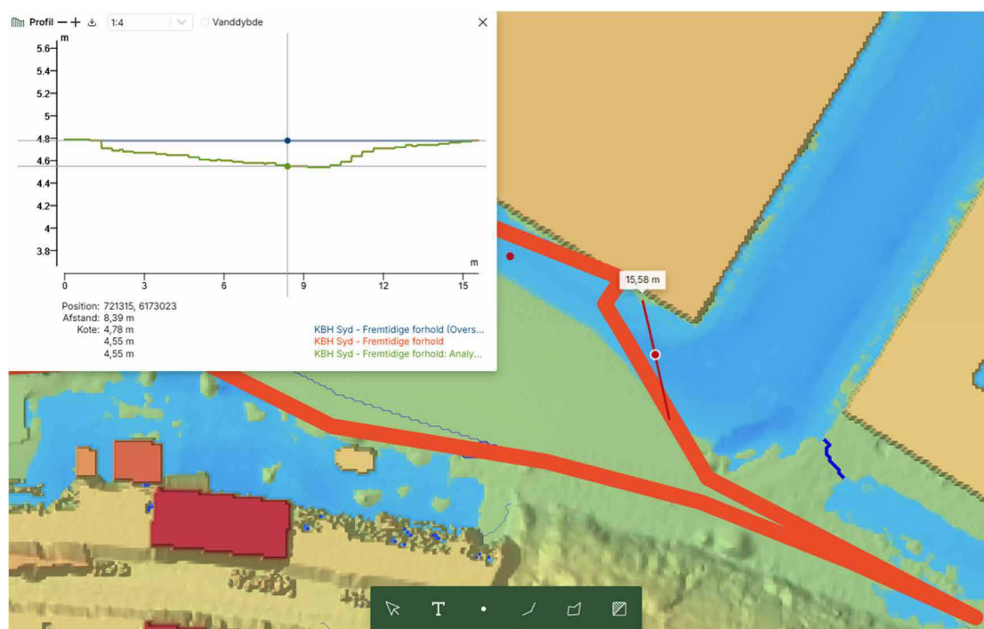
Figur 14 – Kote for afstrømning ud af området
