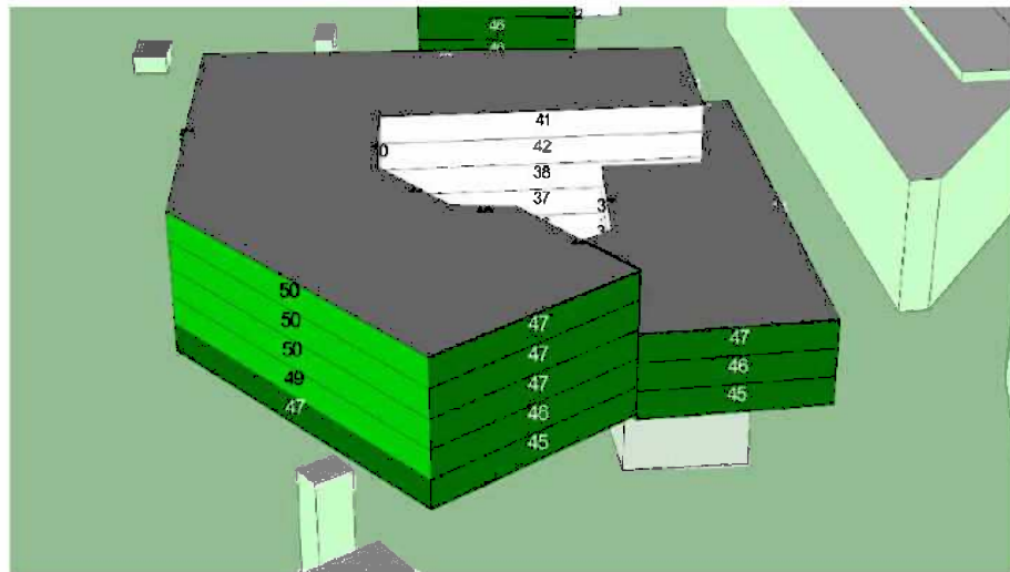
Figur 12: Beregnet vejstøjbelastning L_{den} i dB, Byggefelt 1, set fra syd.
