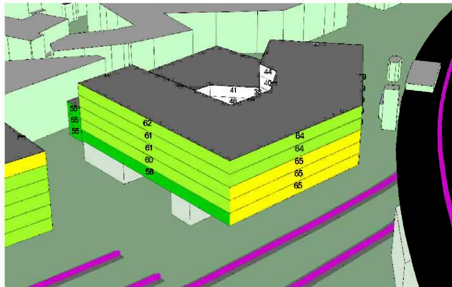
Figur 2: Beregnet jernbanestøj L_{den} i dB, Byggefelt 1 (kontor), set fra vest.
