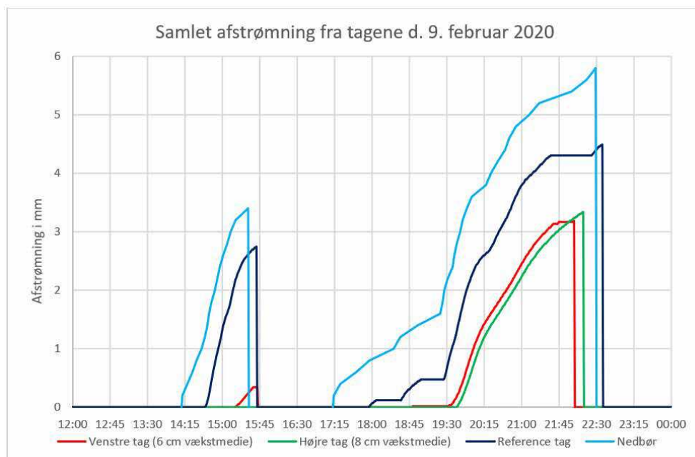
Figur 5-1 Afstrømning og nedbør fra en hændelse i februar 2020.
