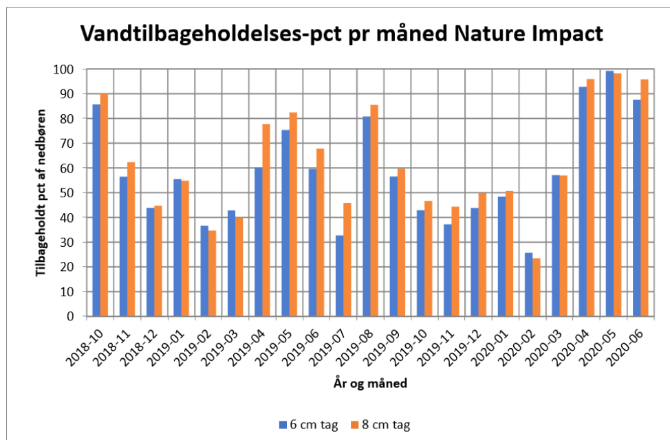
Figur 3-7 Vandtilbageholdelsen på månedsbasis
