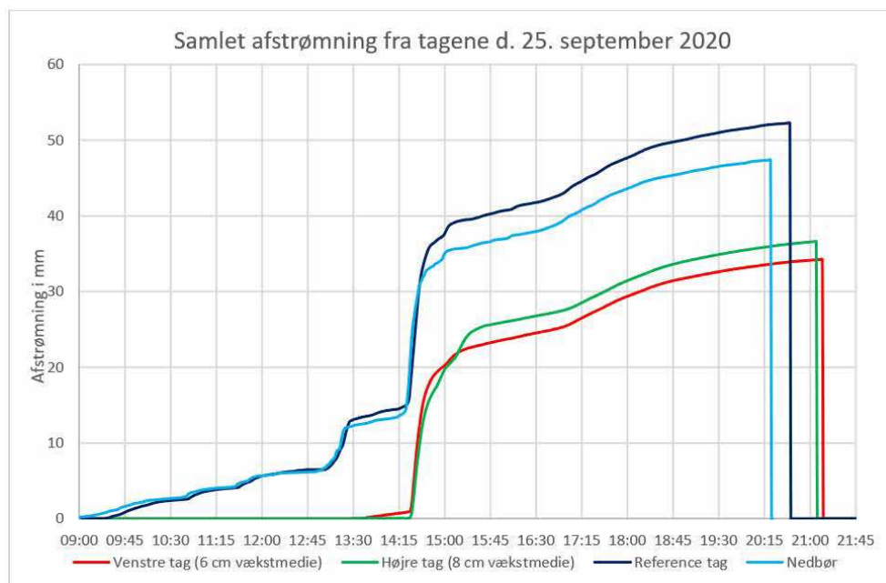
Figur 4-1 Summeret nedbør og afstrømning i forbindelse med skybrud i Lyngby-Taarbæk d. 25. september 2020.
