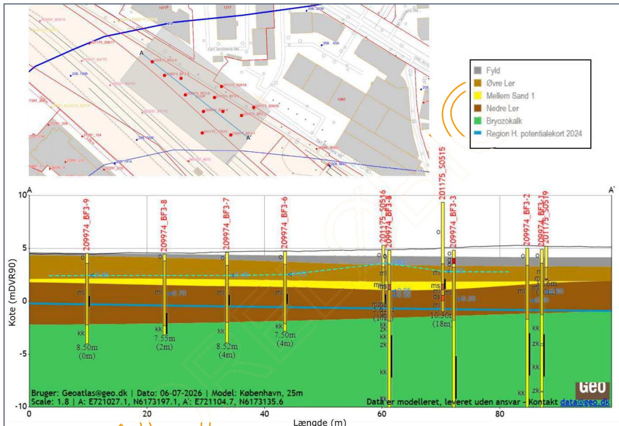
Figur 1.2: Geologisk profil fra GeoAtlas Live med borer og pejlinger vist. Det terrænnære grundvandspejl er markeret med turkis stiplede linje. Det forventede potentiale for det primære grundvandspejl er vist med blå linje.
