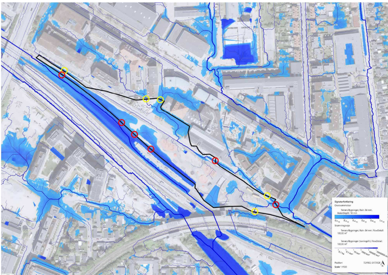
Figur 7 – Scalgoanalyse ekstremregn, strømningsveje eksisterende forhold
