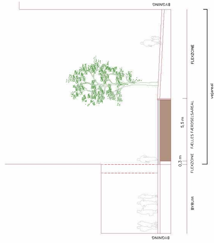
Snit C-C
