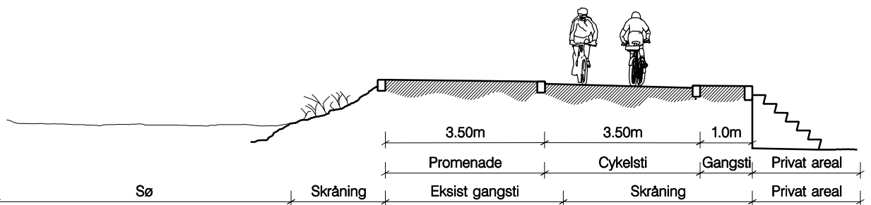
Principalsnit i strækning type C2
