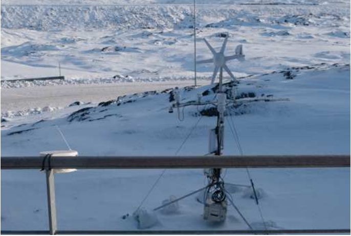
Første version af sensor-instrument (SCK - Temperature, Humidity, Noise, Air quality (CO2), Light, Barometric pressure) i dialog med GEUS semi-stationære vejrstation, 3D-printet (Nuuk, november 2024). Foto: Gudrun Havsteen-Mikkelsen.
