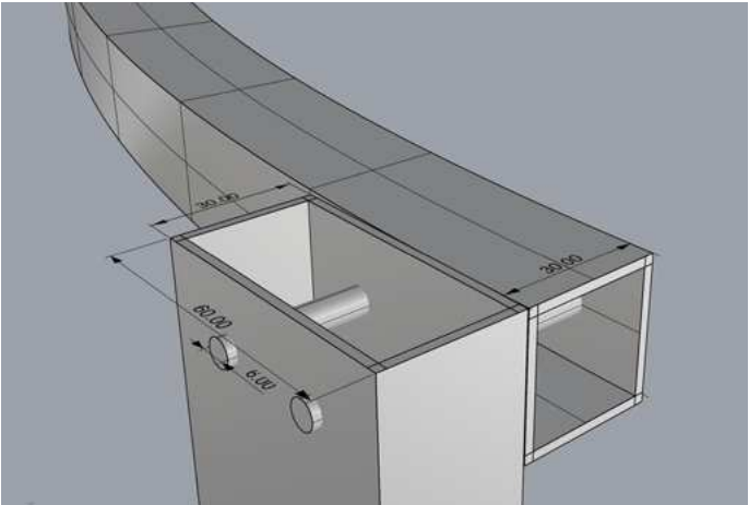
Teknisk skitse af metal-konstruktion. Sensorinstrumentets struktur (en simulerende arktisk vejrstation) er fremstillet af aluminiumsprofiler i målene 30x30 mm. Rendering: Gudrun Havsteen-Mikkelsen.
