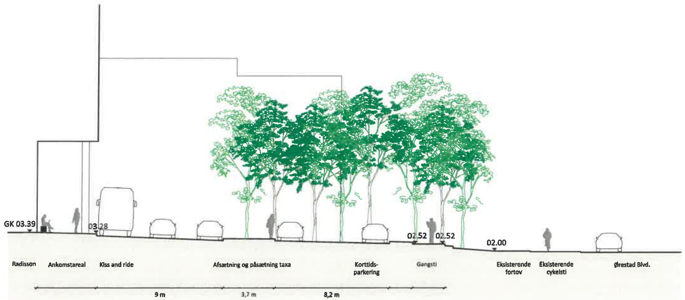
Snit B-B - Vejtype b - Forplads set mod nord
