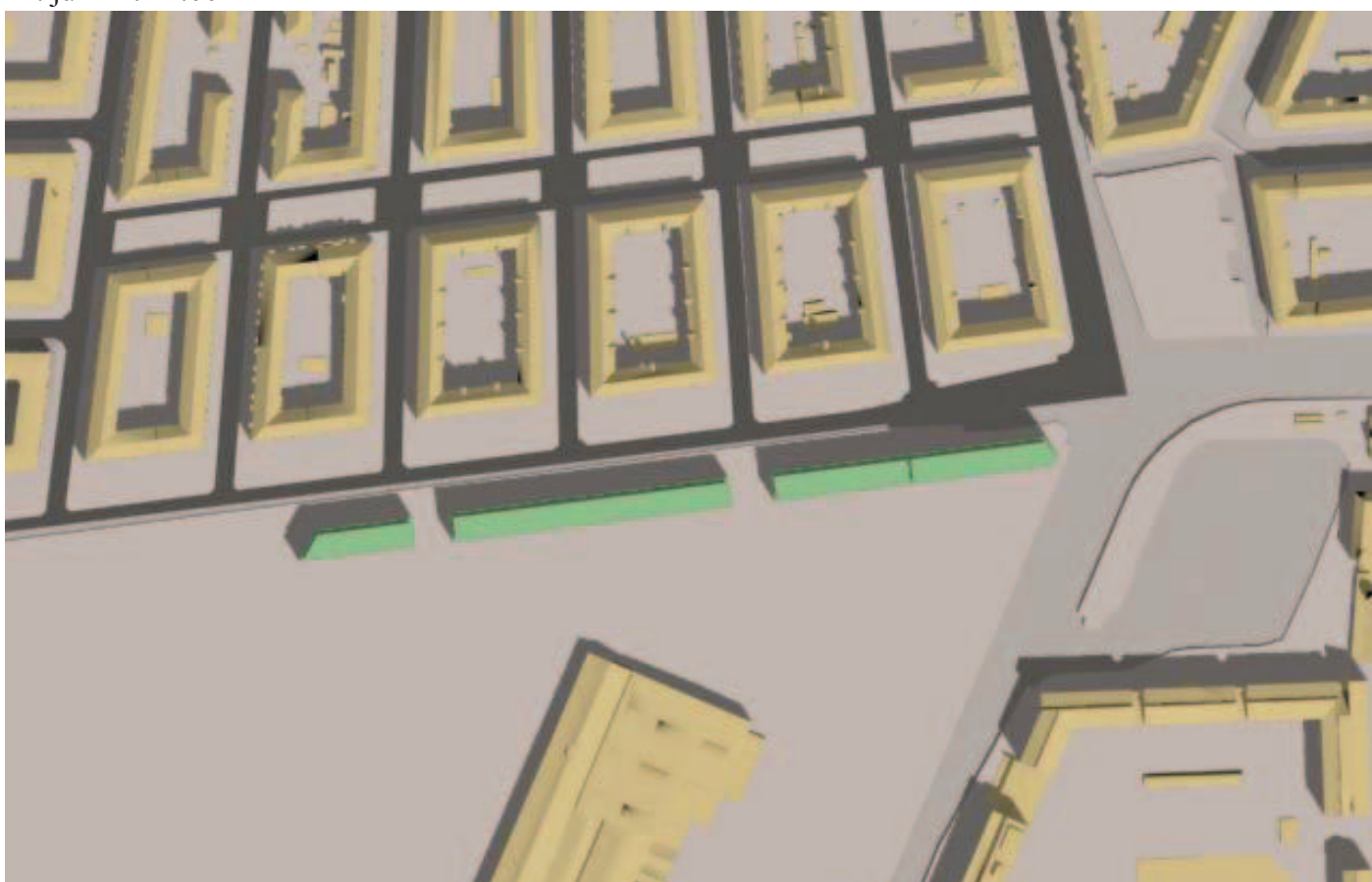
21. juni kl. 12.00
