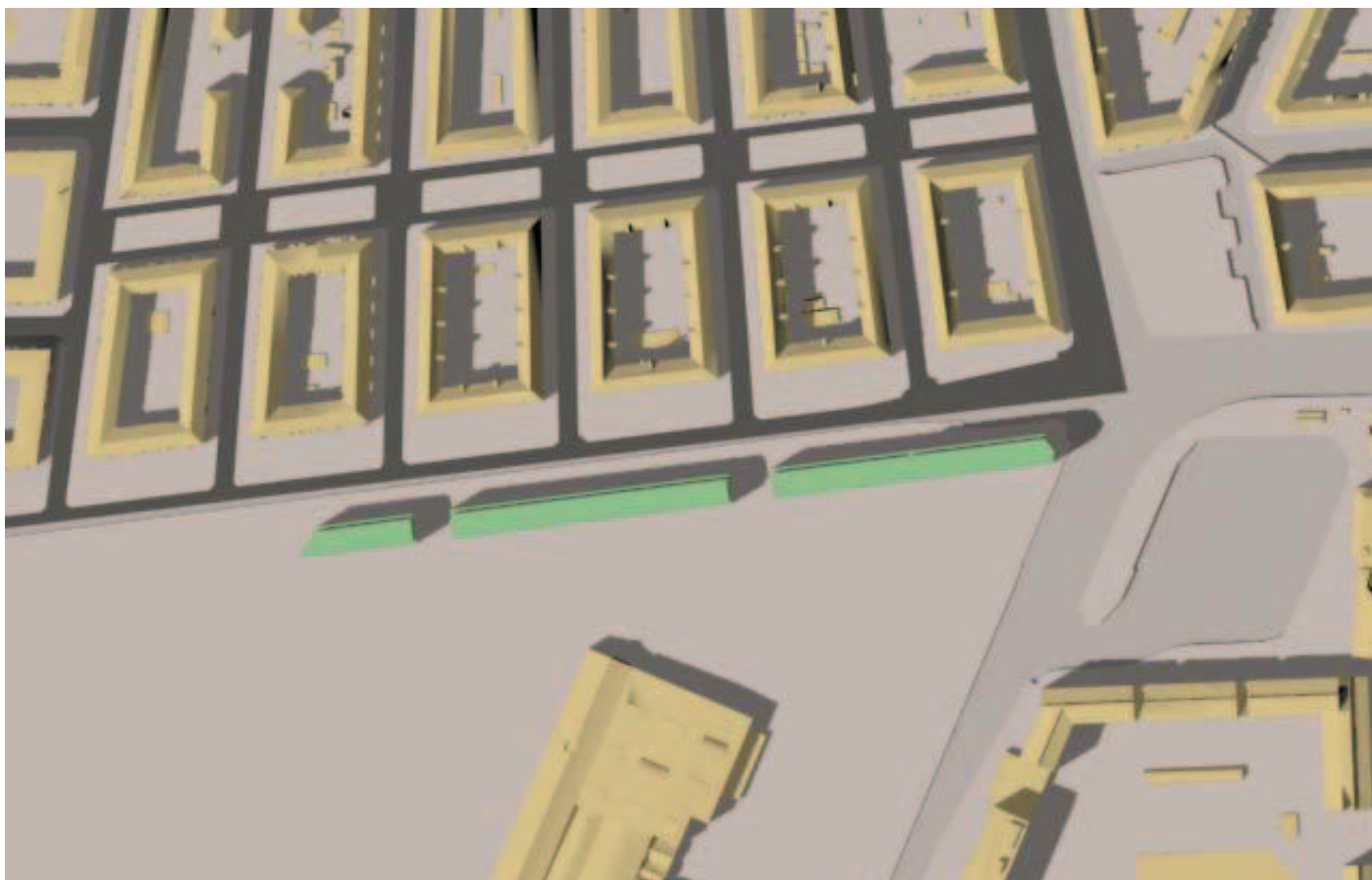
21. juni kl. 16.00
