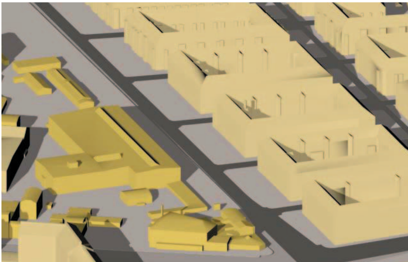
21. marts kl. 9.00
