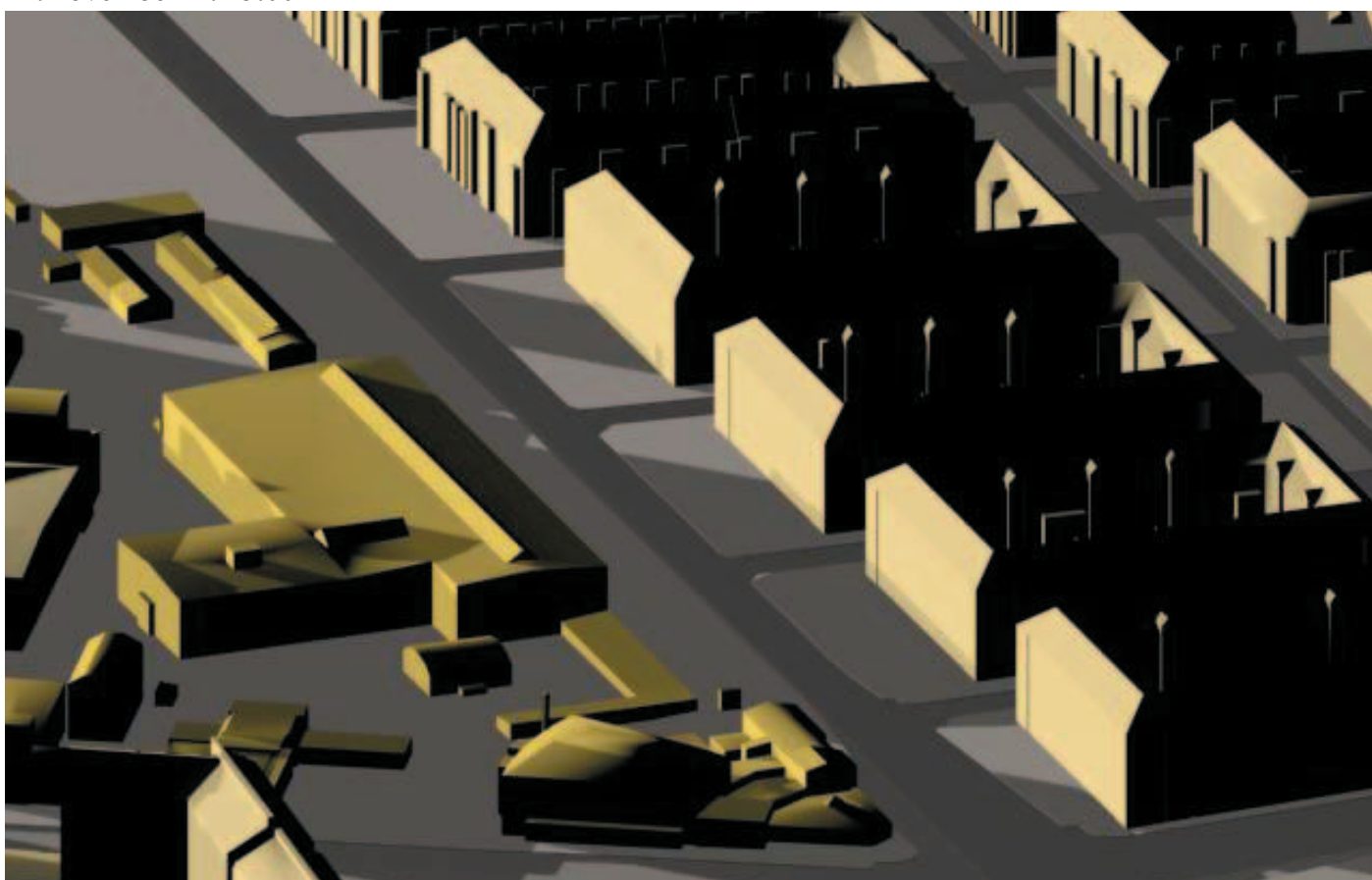
21. november kl. 15.00
