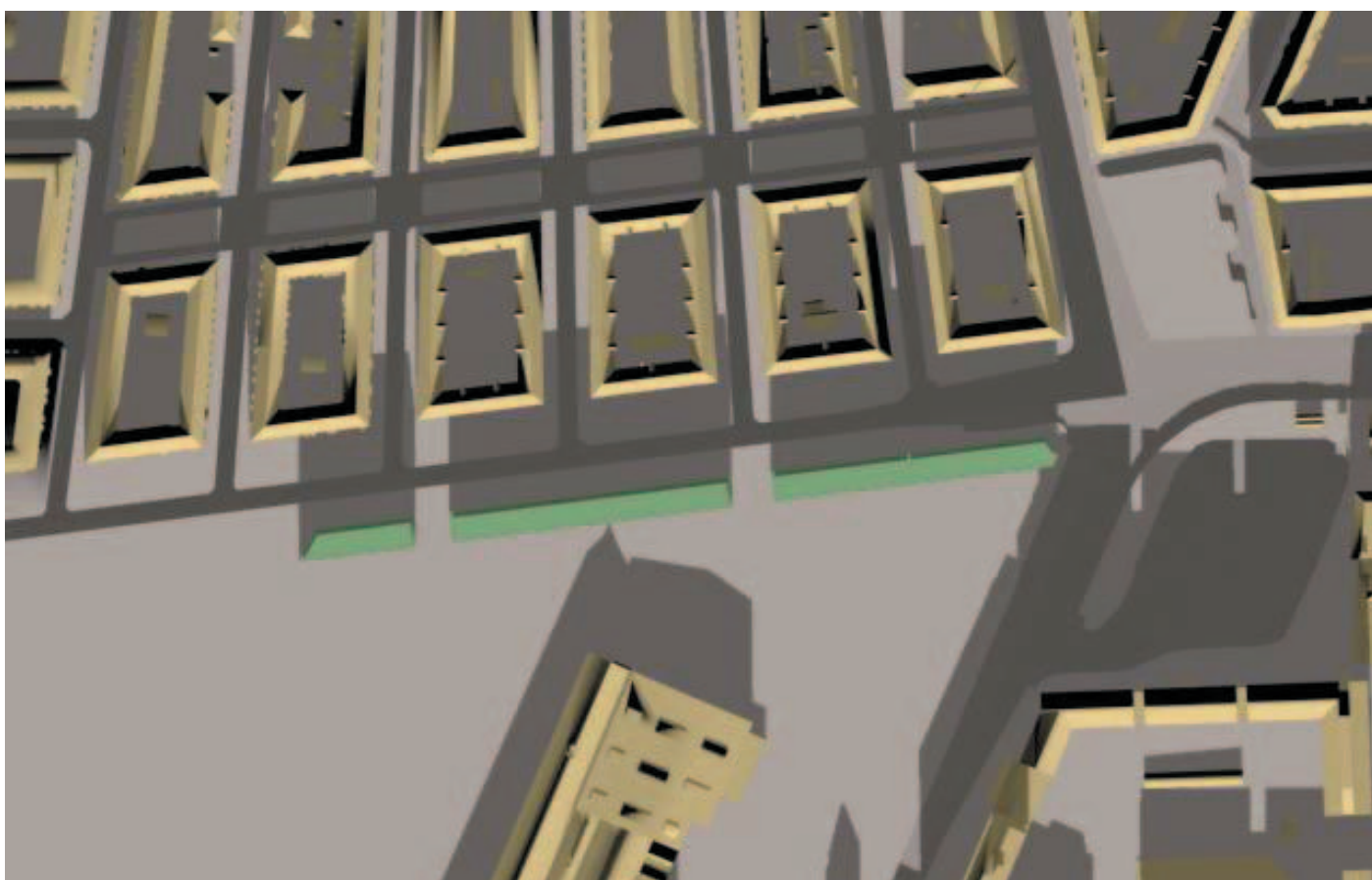
21. november kl. 12.00
