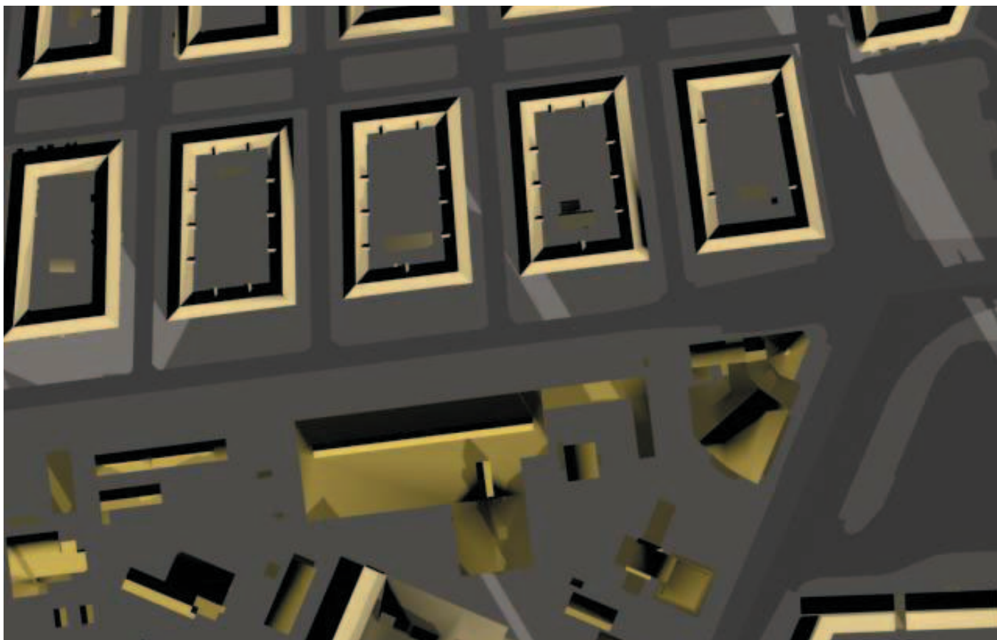
21. december kl. 10.00
