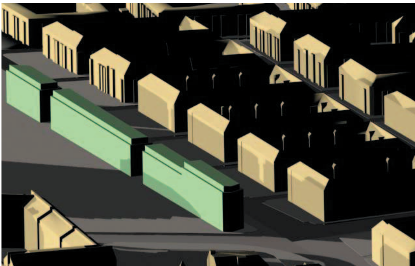
21. december kl. 15.00
