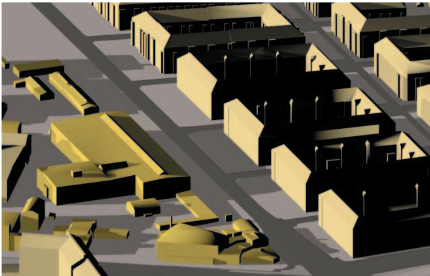
21. december kl. 13.00
