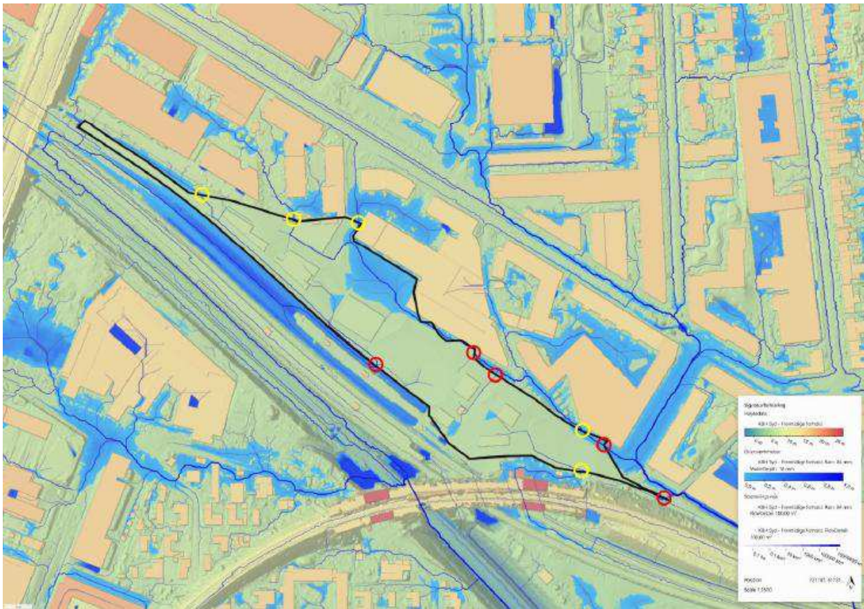
Figur 19.3: Scalgoanalyse af ekstremregn ved højdemodel/situationsplan af d. 21. maj 2026. De gule cirkler angiver strømningsveje ind i projektområdet, mens den røde cirkler angiver strømningsveje ud af projektområdet /Bilag 9/.
