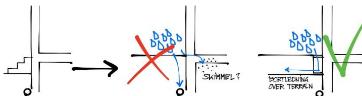
Figur 19: Eksempel hvor trin udignes til niveaufri adgang, og hvor der sørges for, at facadevand ledes bort over terræn – ikke nedsives til omfangsdræn eller fugtfølsom sokkel.
