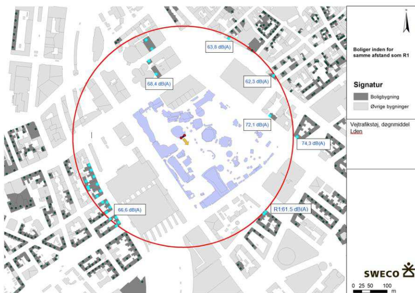
Figur 11-1 Vejstøjtrafik, årsdøgnsmiddel ( L_{den} ) ved boliger, der ligger i samme og kortere afstand til Plæns scene som referenceposition R1, Stoltenberggade 1 4 .
