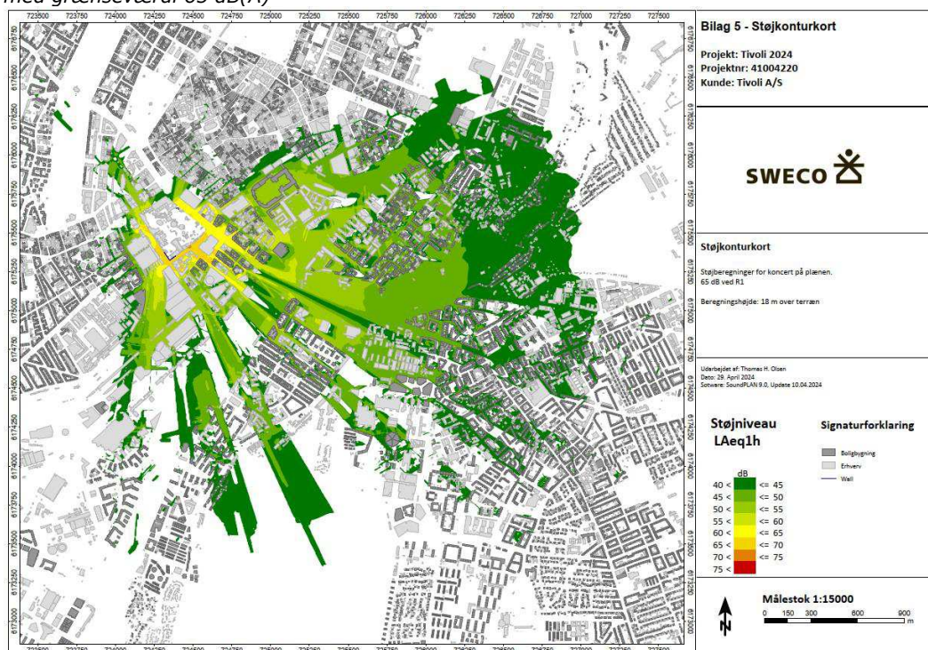
Figur 9-8 Støjudbredelse 18 m over terræn ved afholdelse af koncerter på Plænen med grænseværdi 65 dB(A)
