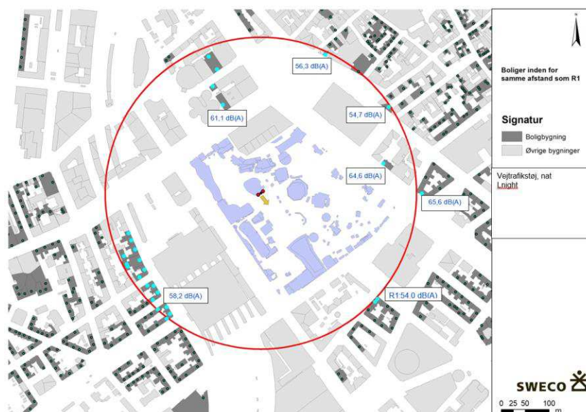
Figur 11-2 Vejstøjtrafik, nat ( L_{night} ) ved boliger, der ligger i samme og kortere afstand til Plæns scene som referenceposition R1, Stoltenberggade 1 4 .
