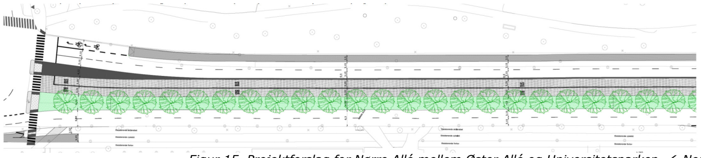
Figur 15. Projektforslag for Nørre Allé mellem Øster Allé og Universitetsparken. ← Nord
