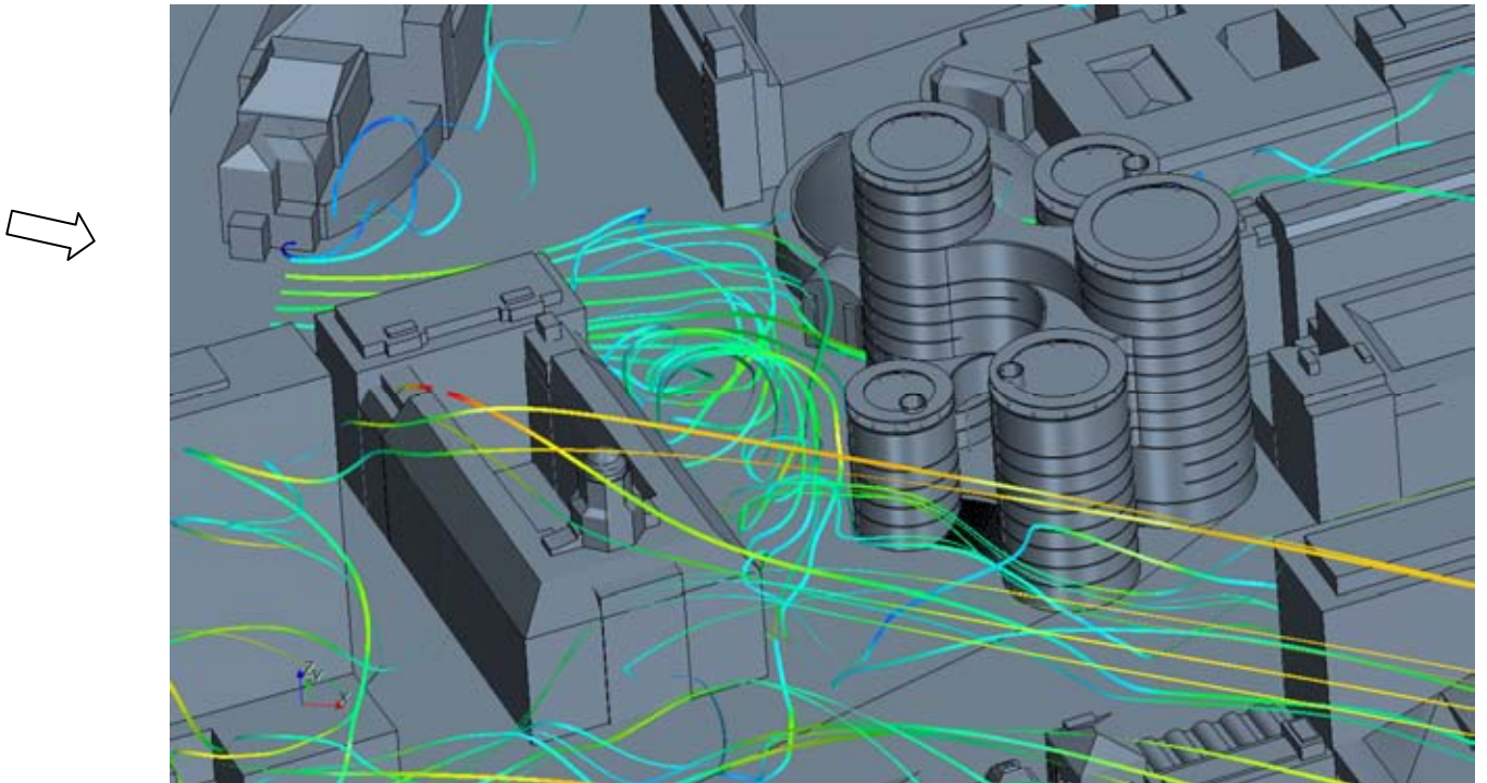
Figur 6.1 Strømlinjer. Vestenvind.
