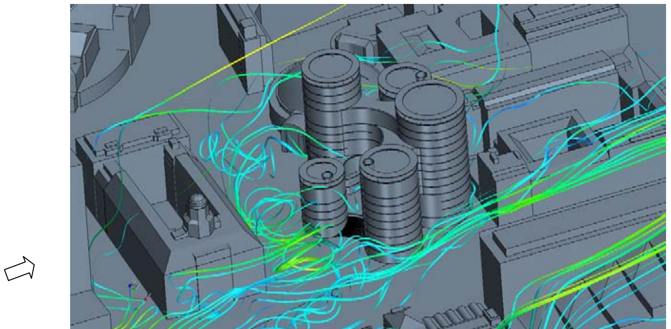
Figur 6.2 Strømlinjer. Sydvestenvind.
