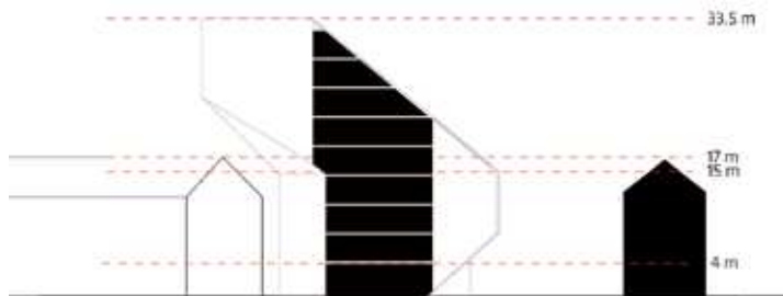
Snit A-A
