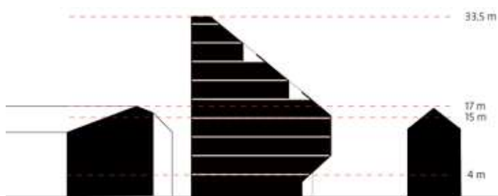
Snit D-D
