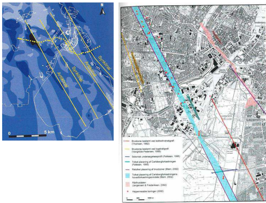
Fig. 12. Forfatterens bud på placering af Carlsbergforkastningens hovedforastningsområde samt brudlinier, herunder retolkede. Bemærk Rådhusdalens orientering i forhold til Carlsbergforkastningens.
