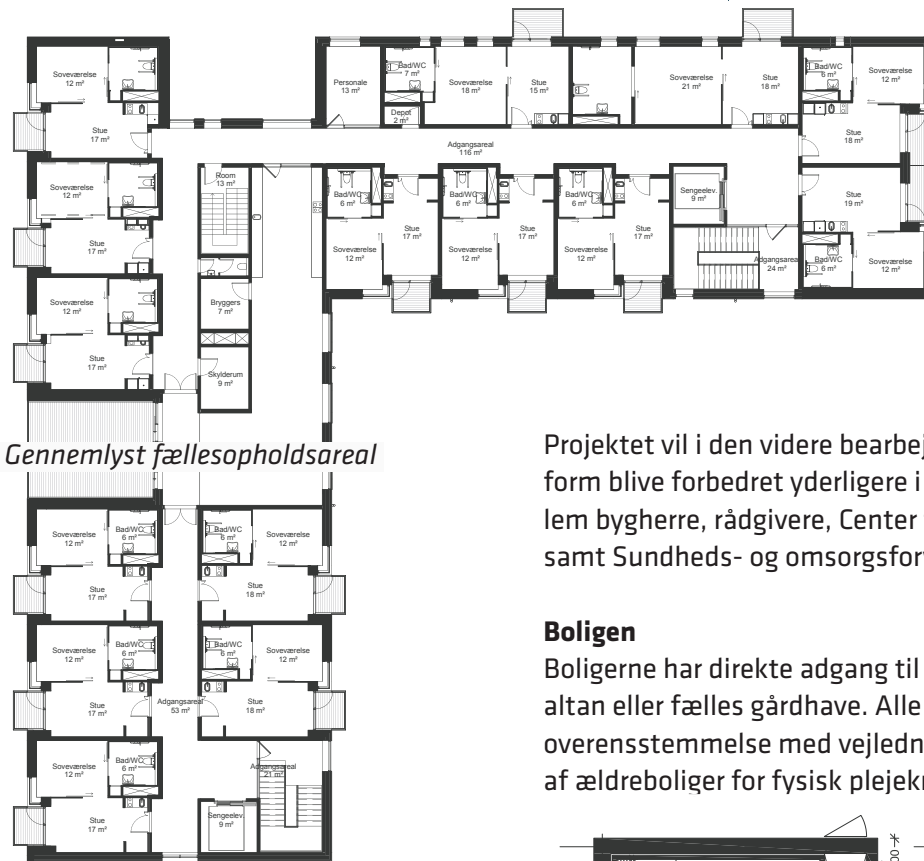
Etageplan
