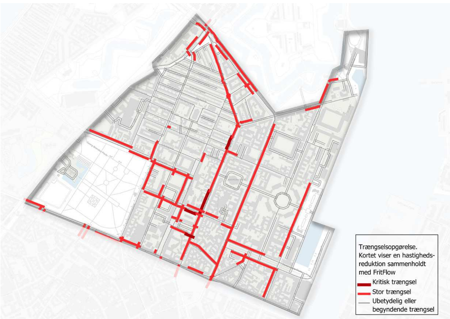
Figur 38 Trængsel i eftermiddagsspidstimen. Kilde: Slangetællinger biltrafik i uge 15 og 16 og GPS-data fra TomTom
