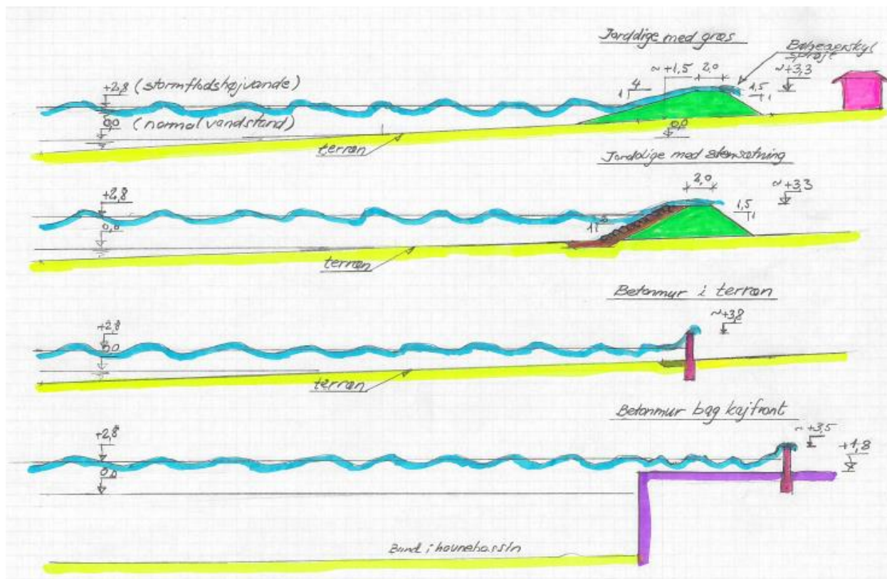
Figur 9-1 Princippet for bølger, der rammer et dige eller lodret mur og det resulterende bølgeoverskyl.
