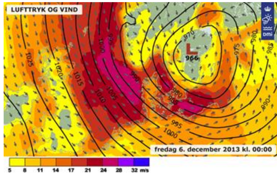
Figur 8-1 Vejrkort fra stormen Bodil d. 6. december 2013 kl. 00.00.
