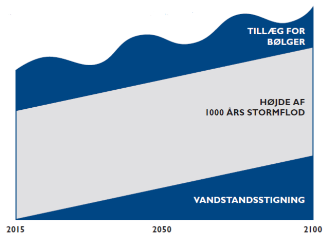
Figur 5 Principiell tegning af sammensætning af beregning for sikringsniveau (Stormflodsplan for København, 2017)
