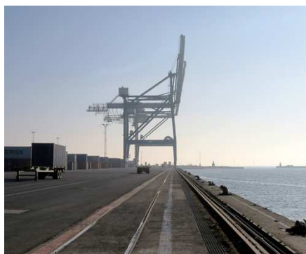
Kranspor og fortøjningspullerter langs den sydlige kajkant.
