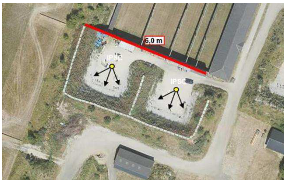
Figur 13-3 - Støjdæpende foranstaltning Bane 14-15, /XX/
