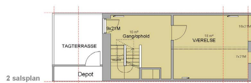
Boligtype 08 - 60 m 2
