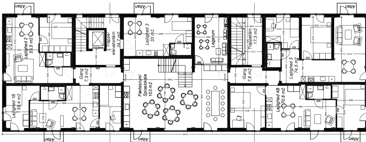
Etageplan 1- 4 sal
