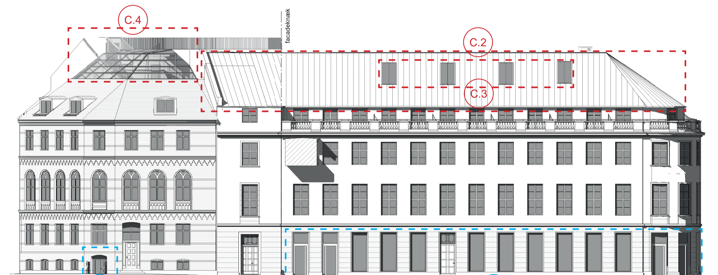
LA06, OPSTALT G 1 : 200
