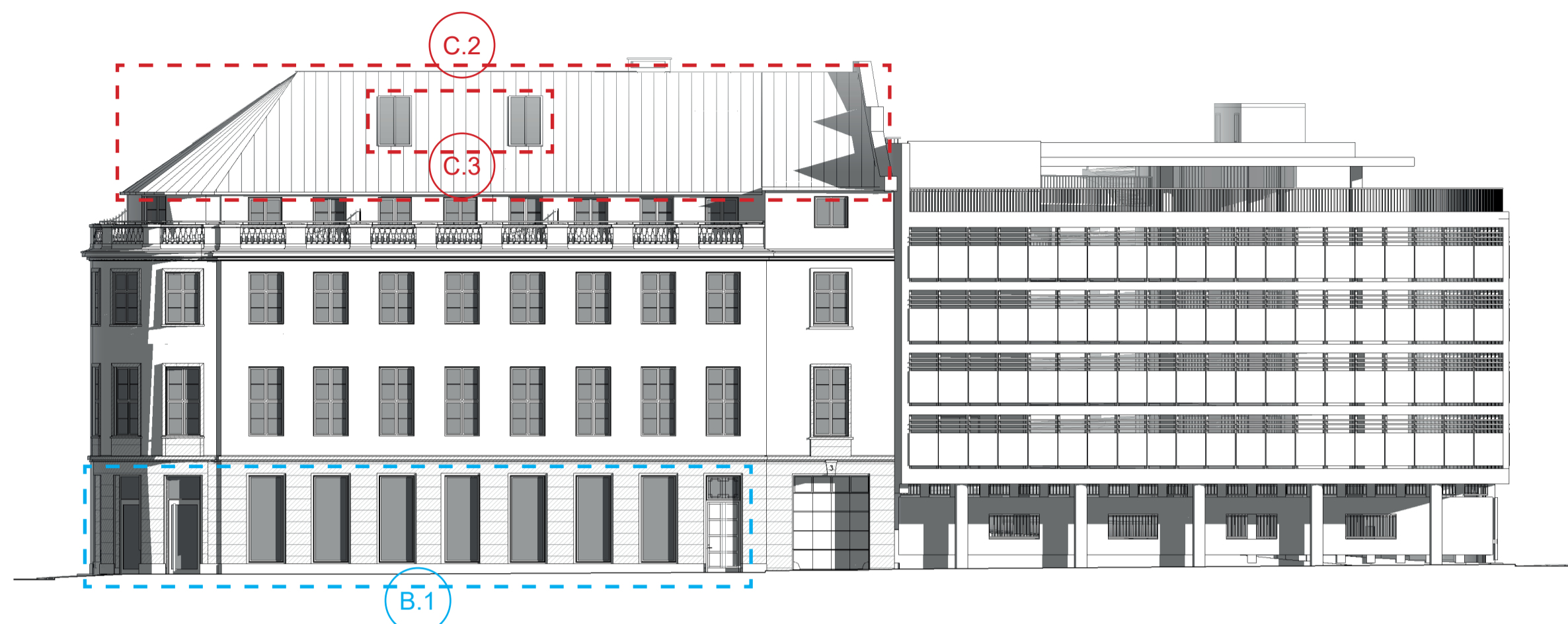
VI03, OPSTALT A 1 : 200
