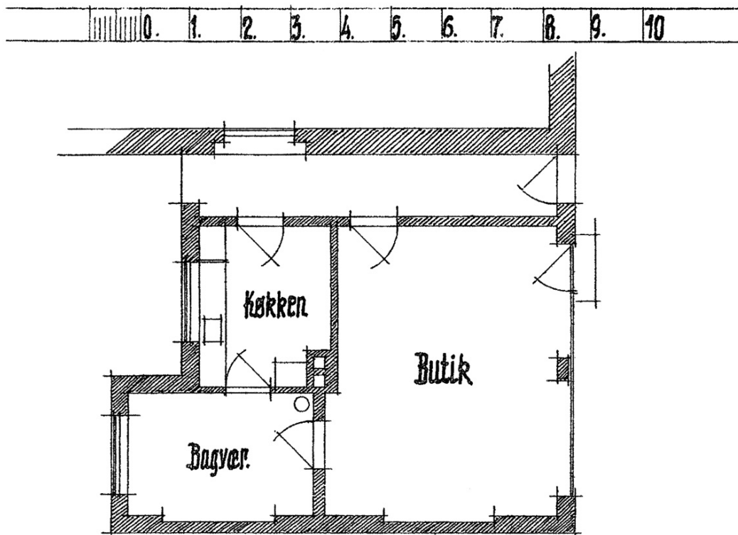
Udsnit af oprindelig plantegning af Arkitekt Frederik Zeuthen
