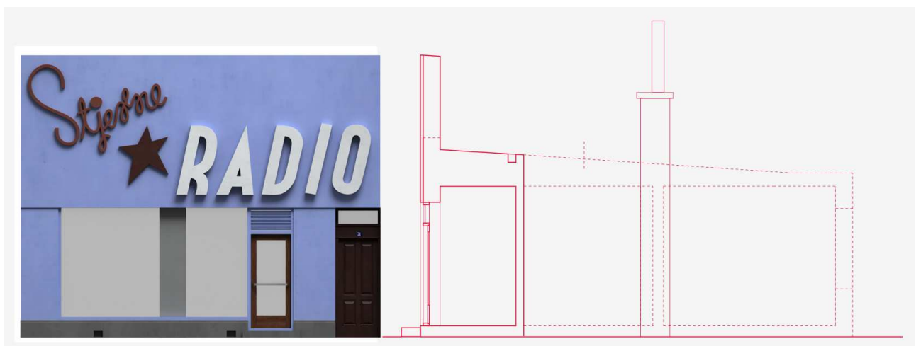
Illustreret facade opstalt og snit. Bygningens oprindelige størrelse ses i snit markeret med stiplet linie.
