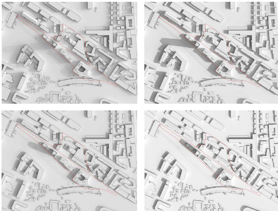
Figur 9.20: Skyggediagrammer for de fremtidige forhold ved sommersonhverv, d. 21. juni. Øverst tv.: Kl. 08.00. Øverst th.: Kl. 09.00. Nederst tv.: Kl. 10.00. Nederst th.: Kl. 11.00. Planområdet er markeret med rød.
