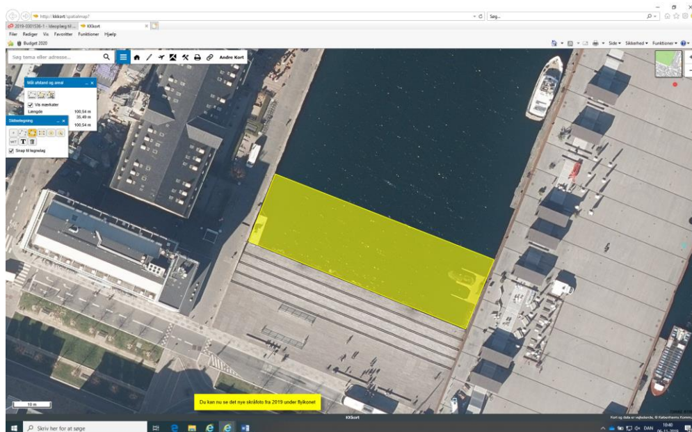
Eksempel på løsning 1 med ca. 65 x 10-20 m badezone på tværs af bassinet.
