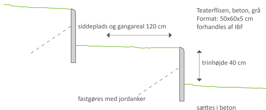
Principielt snit i betonkanter/siddekanter
