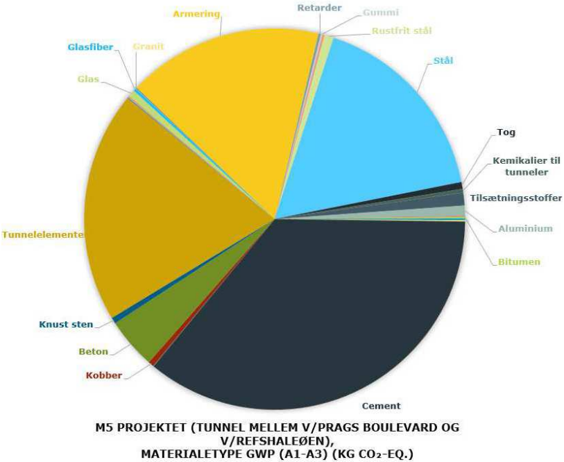
Figur 12.11 Procentvis opdeling af CO 2 e på materialeniveau benyttet i M5 Projektet (Tunnel mellem v/ Prags Boulevard Øst og v/ Refshaleøen).
