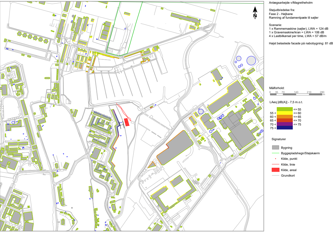
Figur 7.9 Støjudbredelse ved ramning af fundamentpæle til viadukt.
