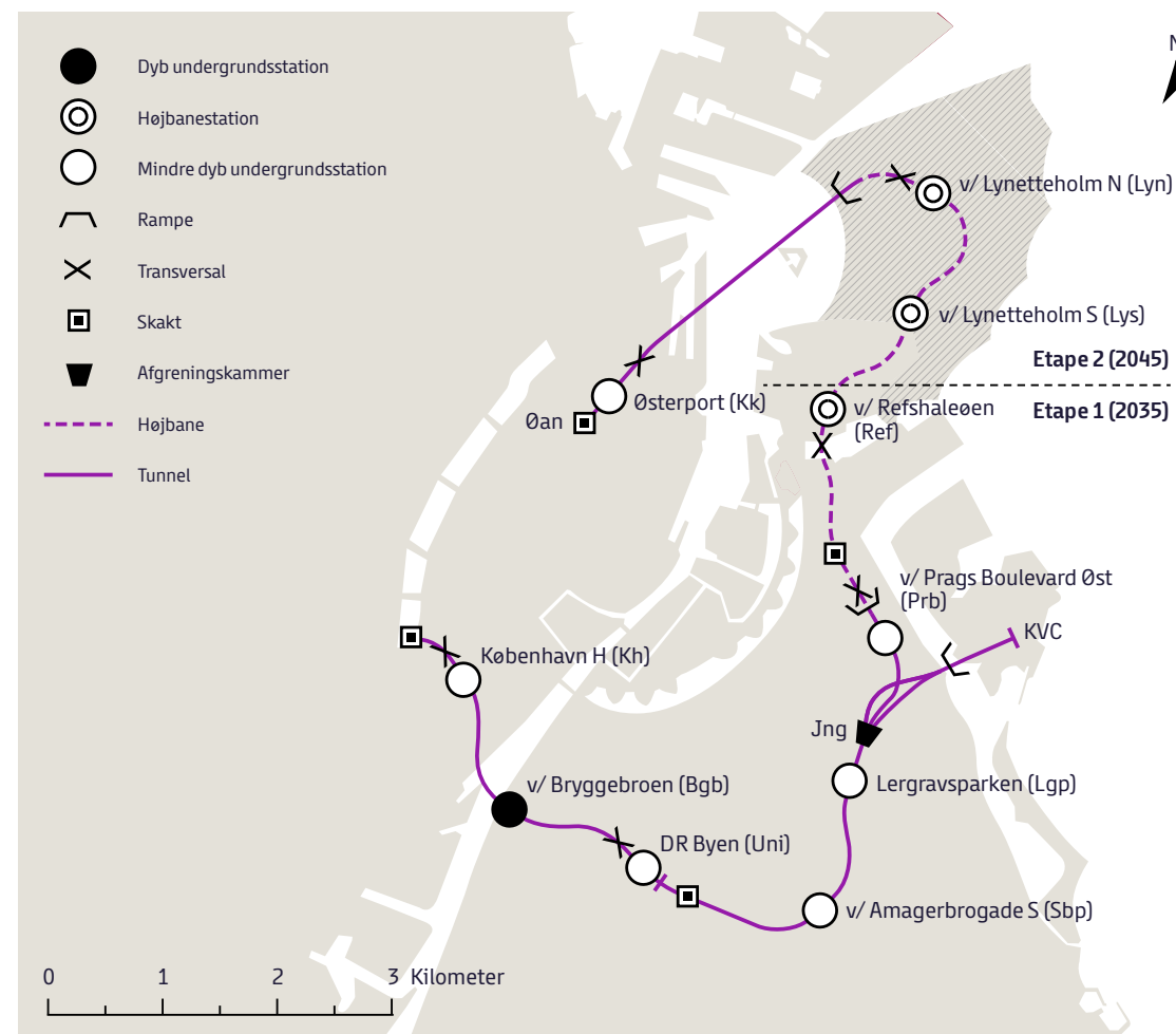
Figur 4.2 Sydlig Løsning for M5.
