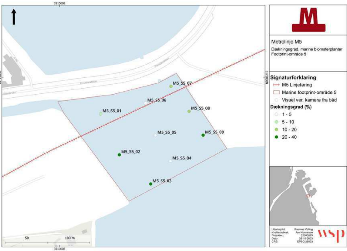
Figur 14.6 Dækningsgrad af marine blomsterplanter i den sydlige del af Prøvestenskanalen baseret på visuel verifikation med håndholdt kamera fra båd. Figur fra (WSP, 2023).
