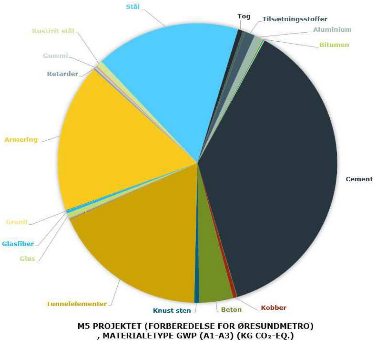
Figur 12.9 Procentvis opdeling af CO 2 e på materialeniveau benyttet i M5 Projektet (Forberedelse for Øresundmetro).
