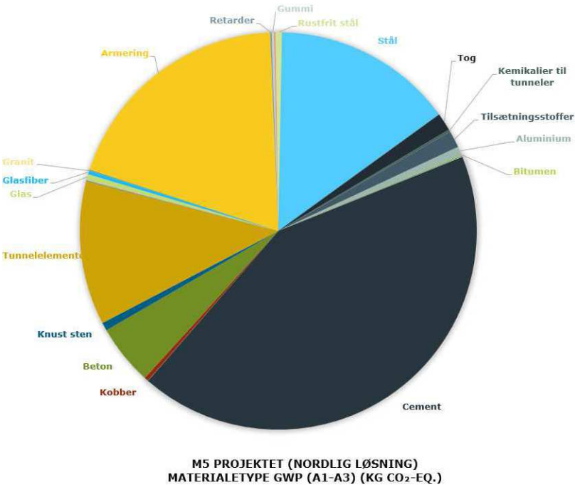
Figur 12.7 Procentvis opdeling af CO 2 e på materialeniveau benyttet i M5 Projektet (Nordlig Løsning).
