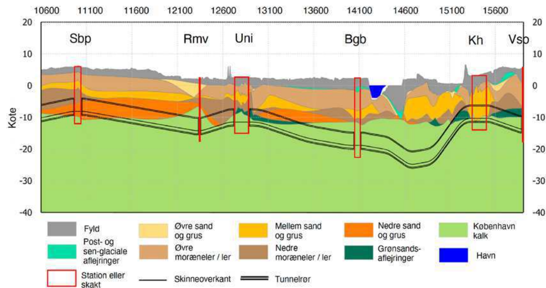
Figur 13.3 Geologisk profil fra Vester Søgade skakt (højre) til v/ Amagerbrogade Syd (venstre). Den sorte linje viser oversiden af skinnerne.
