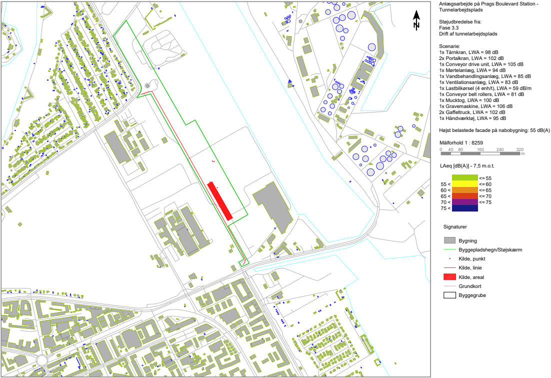
Figur 7.8 Støj kort for Prags Boulevard Tunnelarbejdsplads (PRB), for fase 3.3 ”Drift af tunnelarbejdsplads” som er en fase i døgndrift. Højeste støjniveau beregnet på nærmeste facade er 55 dB.
