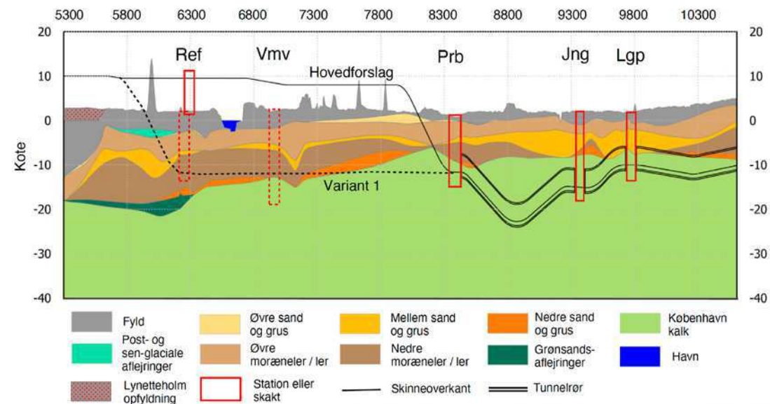
Figur 13.4 Geologisk profil fra Lergravsparken (højre) til den sydlige ende af Lynetteholm (venstre). Den sorte linje viser oversiden af skinnerne.
