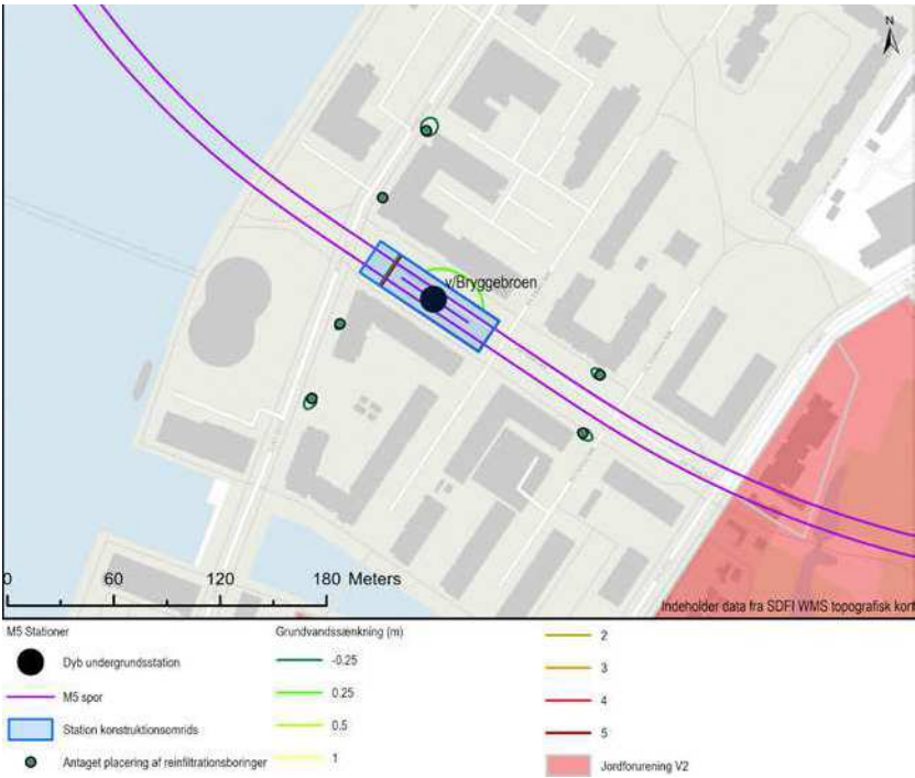
Figur 13.19 Beregnet sænkning i kalkmagasinet ved grundvandssænkning for v/Bryggebroen med vægge til 5 m under bund udgravning og ca. 90 % reinfiltration.
