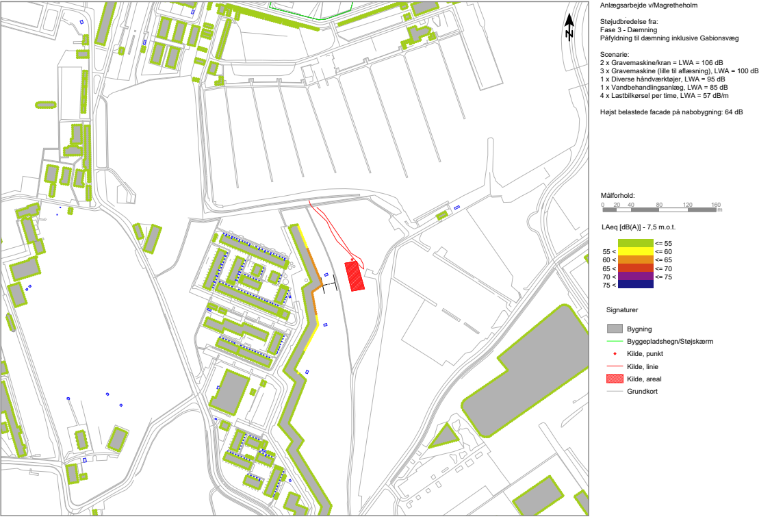
Figur 7.10 Støjudbredelse ved anlæg af dæmning med gabionsvæg.
