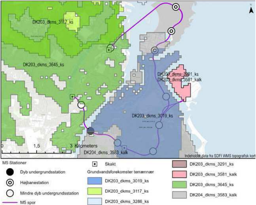
Figur 13.10 Placering af terrænnære grundvandsforekomster.
