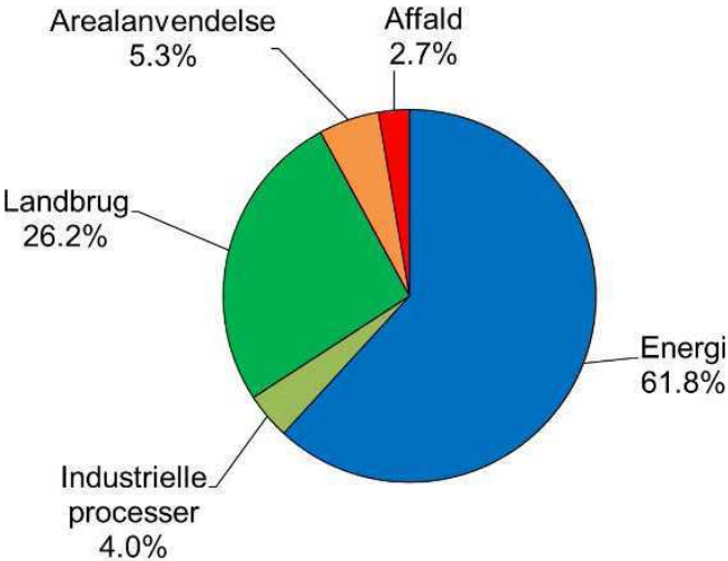
Figur 12.2 Danmarks totale drivhusgasemissioner (CO 2 e) fordelt på hovedsektorer for 2021 (Nielsen et al., 2023).
